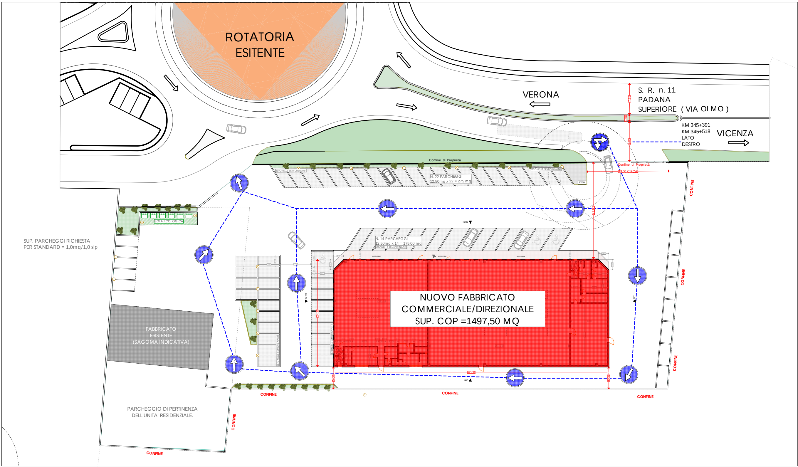
INQUADRAMENTO PIANO TERRA - SCALA 1:500 ● AUTORIZZAZIONE CARRAIO - VENETO STRADE
