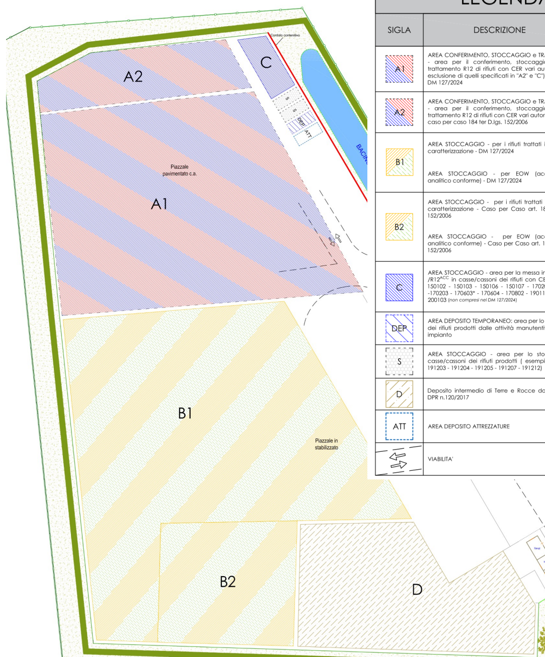
Planimetria generale di impianto (Allegato grafico 1 Layout)
