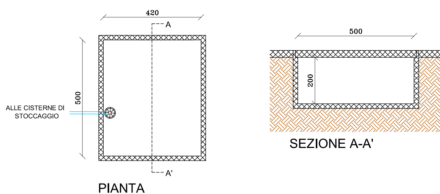
PARTICOLARE VASCA 6 SCALA 1:100
