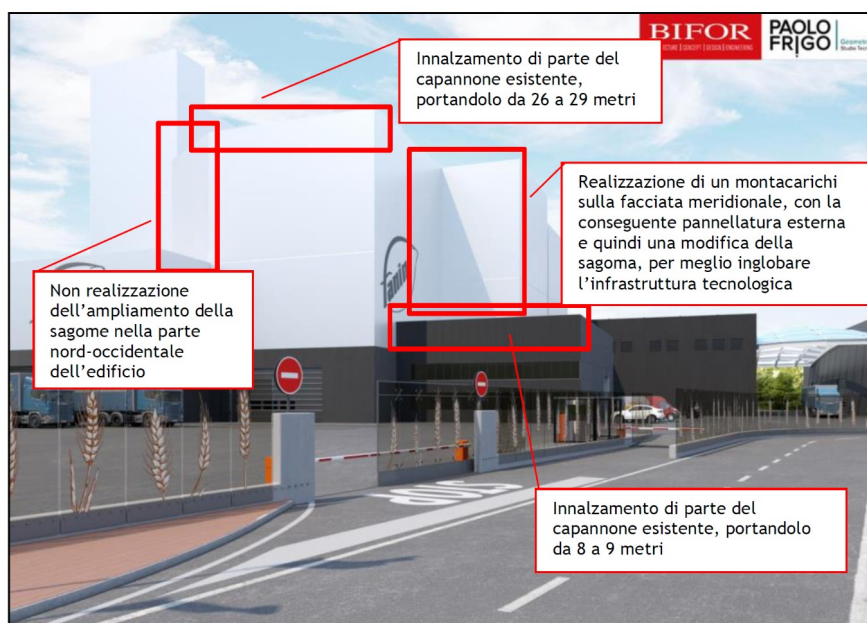
FIGURA 2-32. DEFINIZIONE DELLE MODIFICHE PROPOSTE SU FOTOINSERIMENTO
