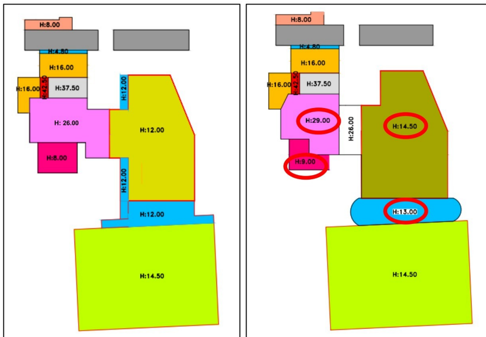
FIGURA 1-1. DIFFERENZE TRA LO STATO DI PROGETTO APPROVATO (SX) E QUELLO DI VARIANTE (DX) IN TERMINI DI PLANIMETRIE E ALTEZZE. SONO EVIDENZIATE LE MAGGIORI DIFFERENZE IN ALTEZZA (CERCHI IN ROSSO)
