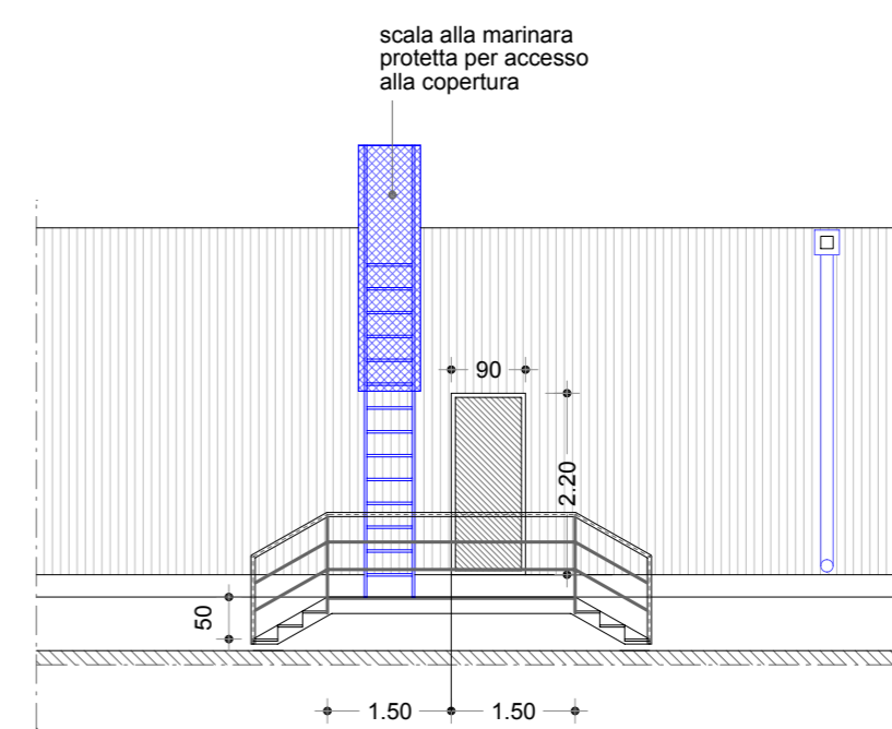
PROSPETTO B-B
