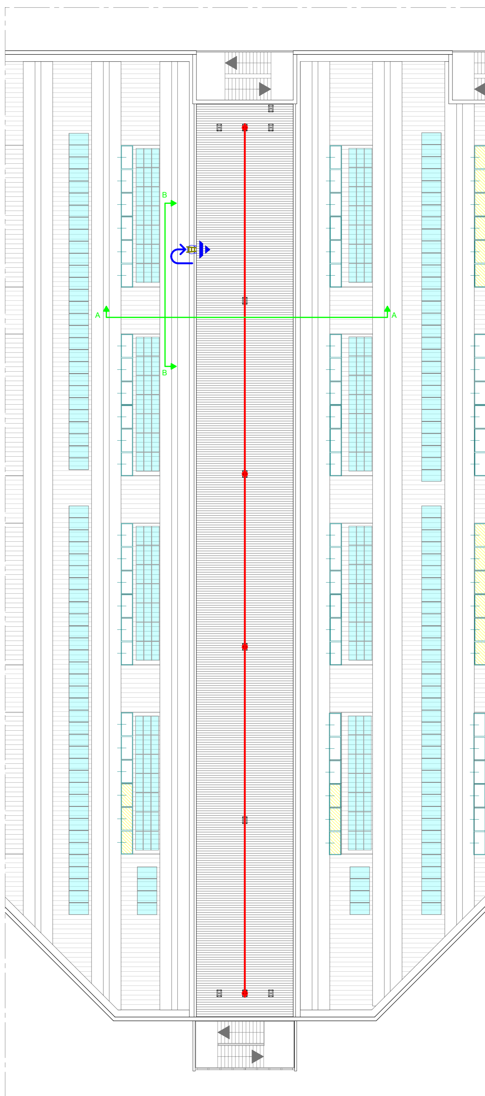
PIANTA LOCALI TECNICI PIANO SECONDO SCALA 1:200
