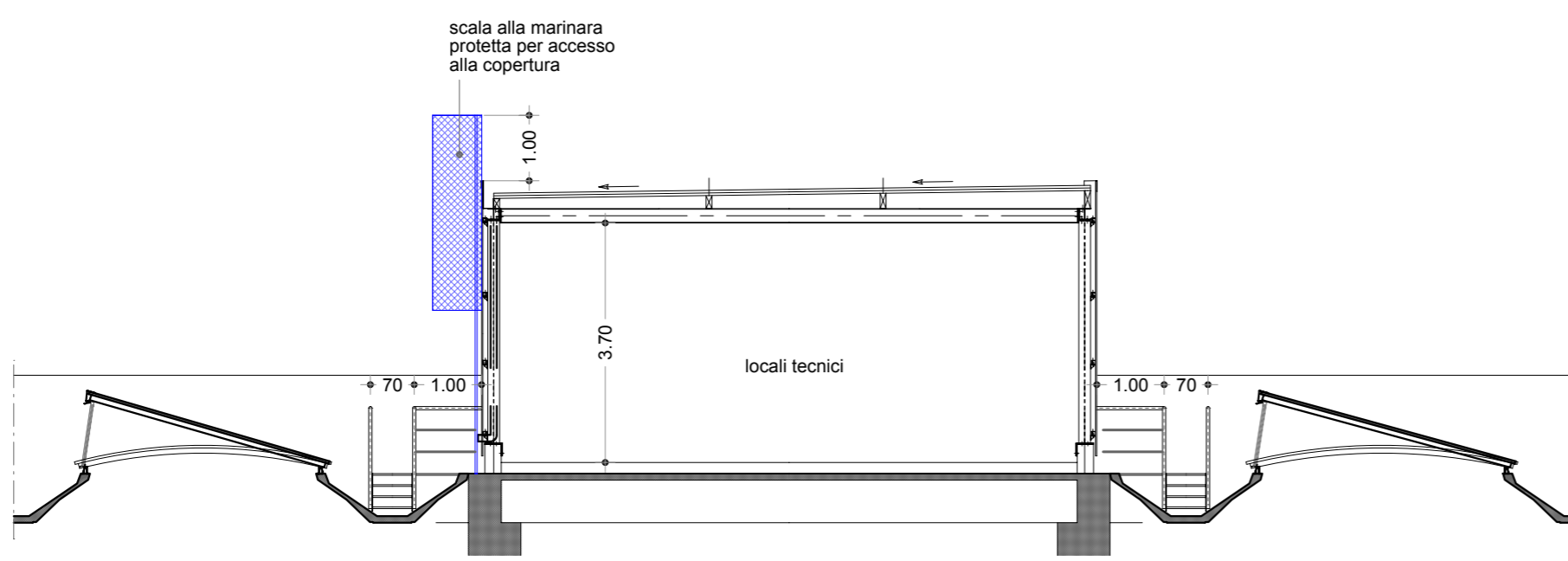
SEZIONE A-A
