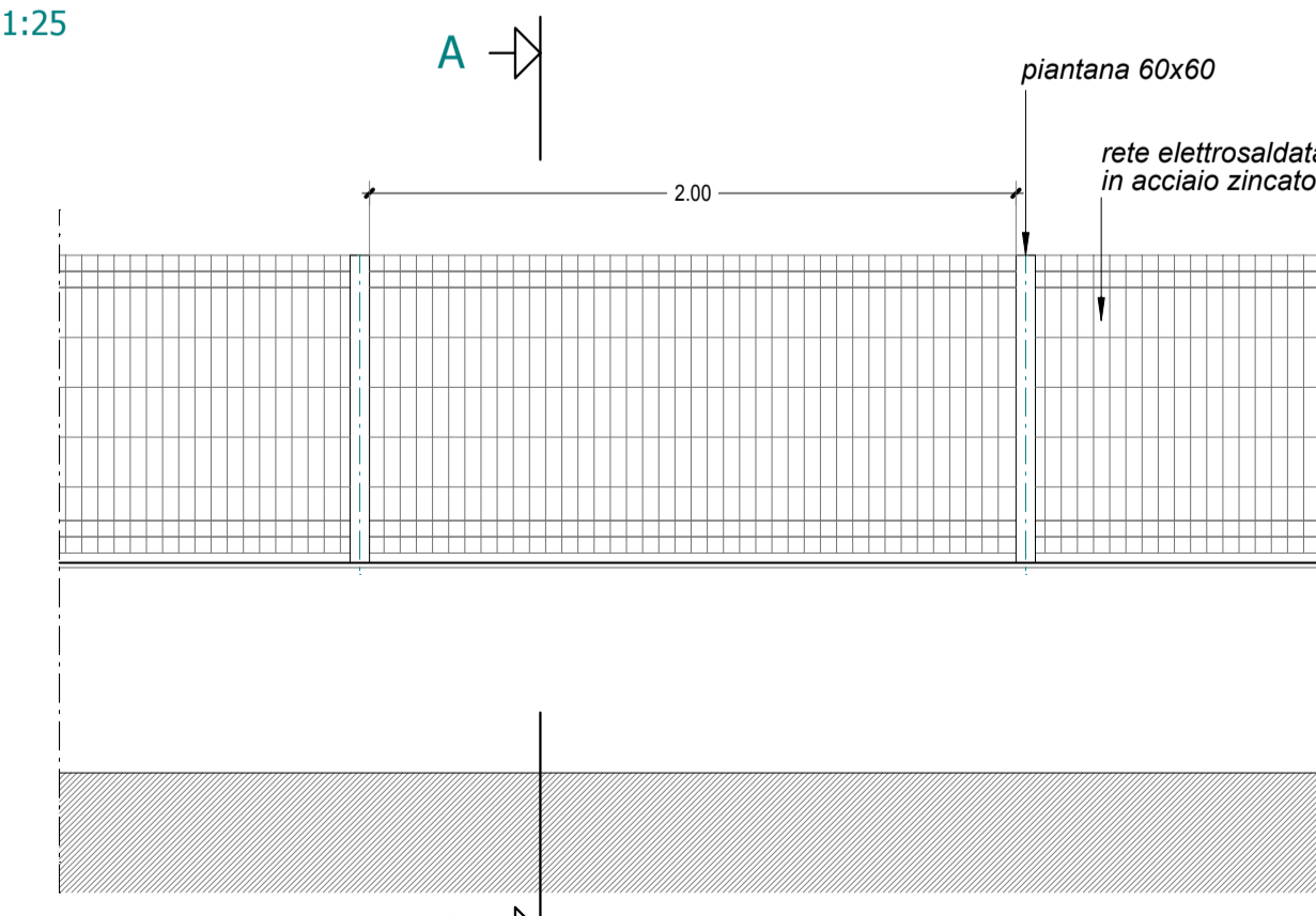
PROSPETTO SU LOTTI CONFINANTI
