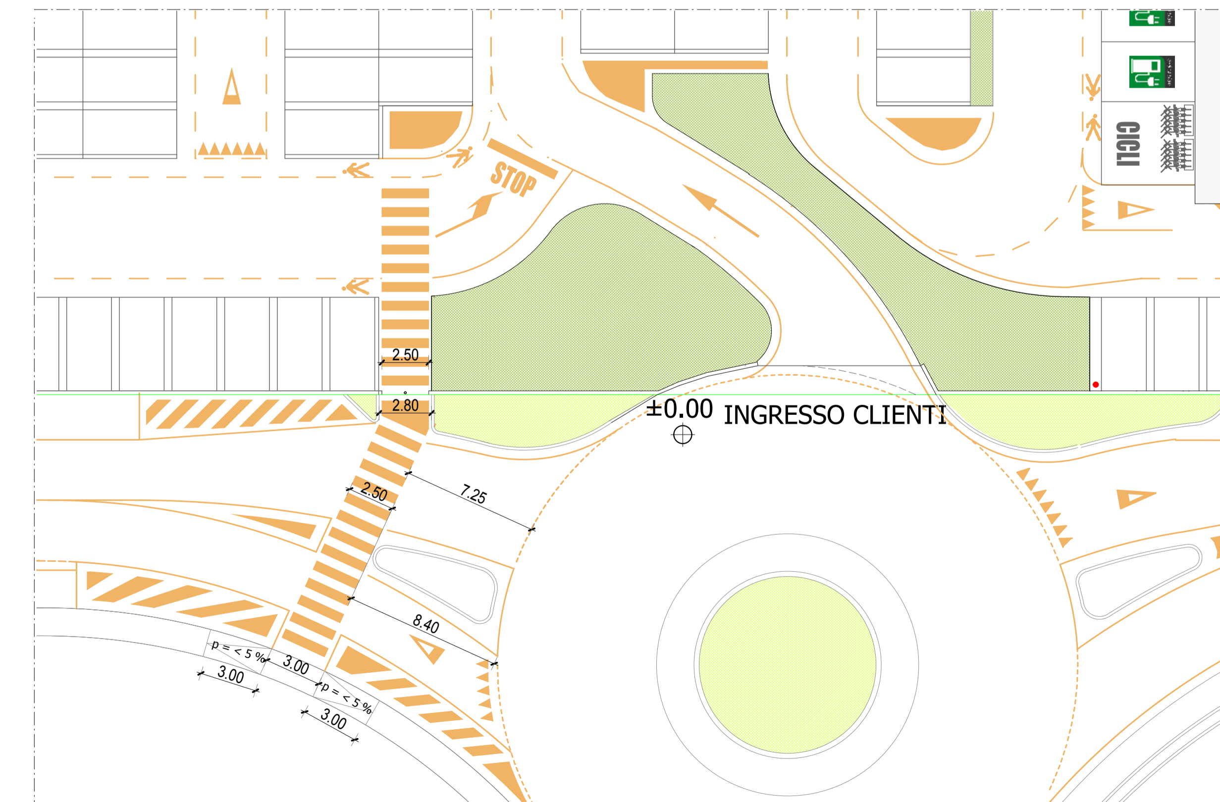
NUOVO INGRESSO PEDONALE
