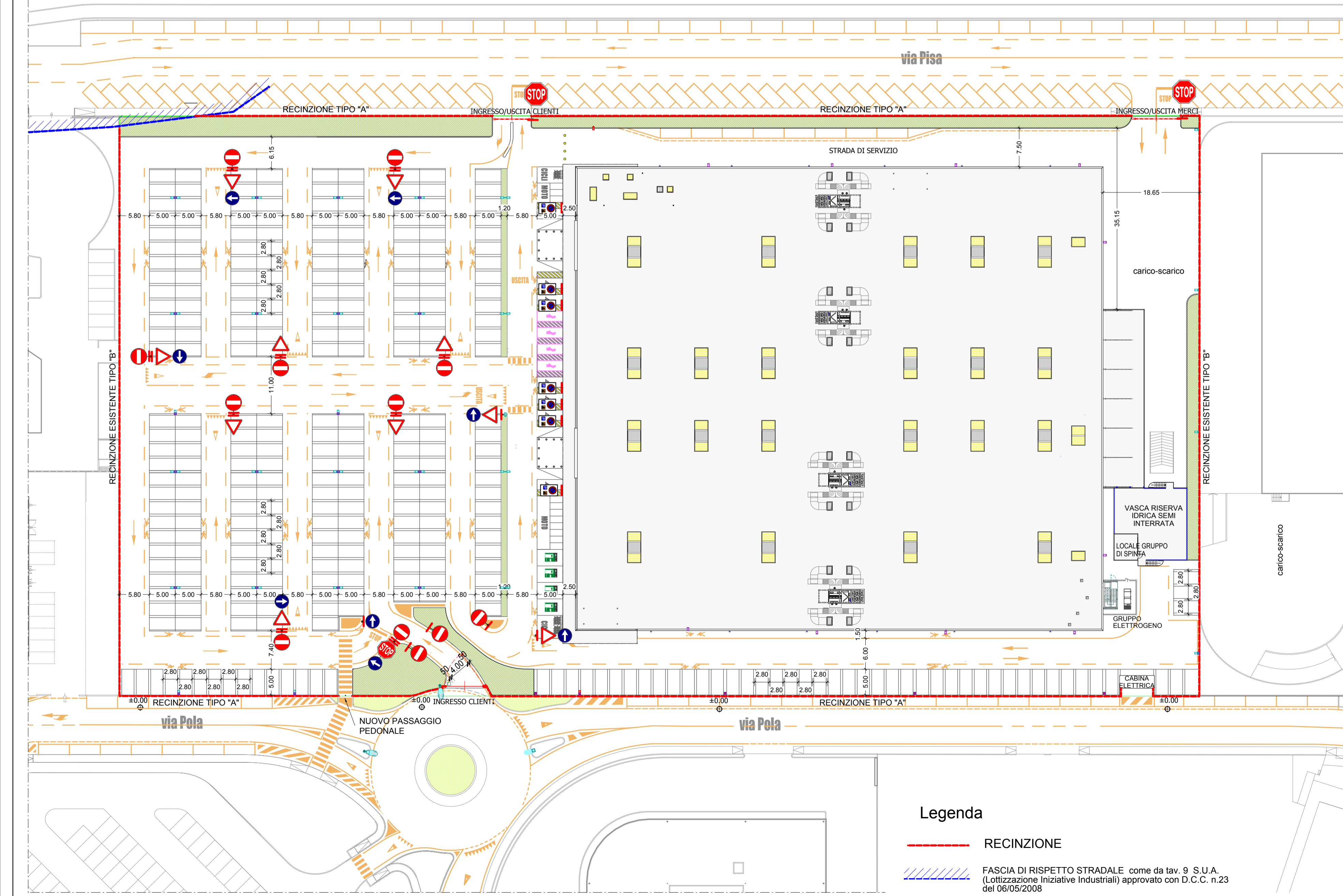
PLANIMETRIA RECINZIONI E PASSI CARRAI - SCALA 1:500
