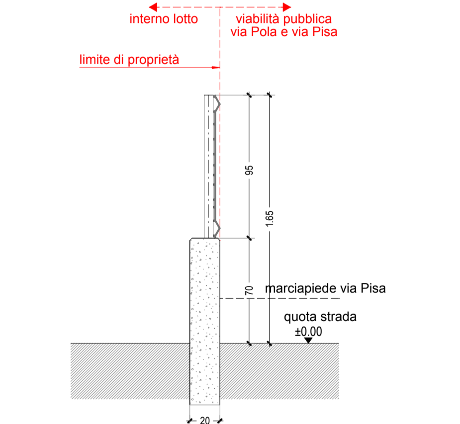
SEZ. A-A
