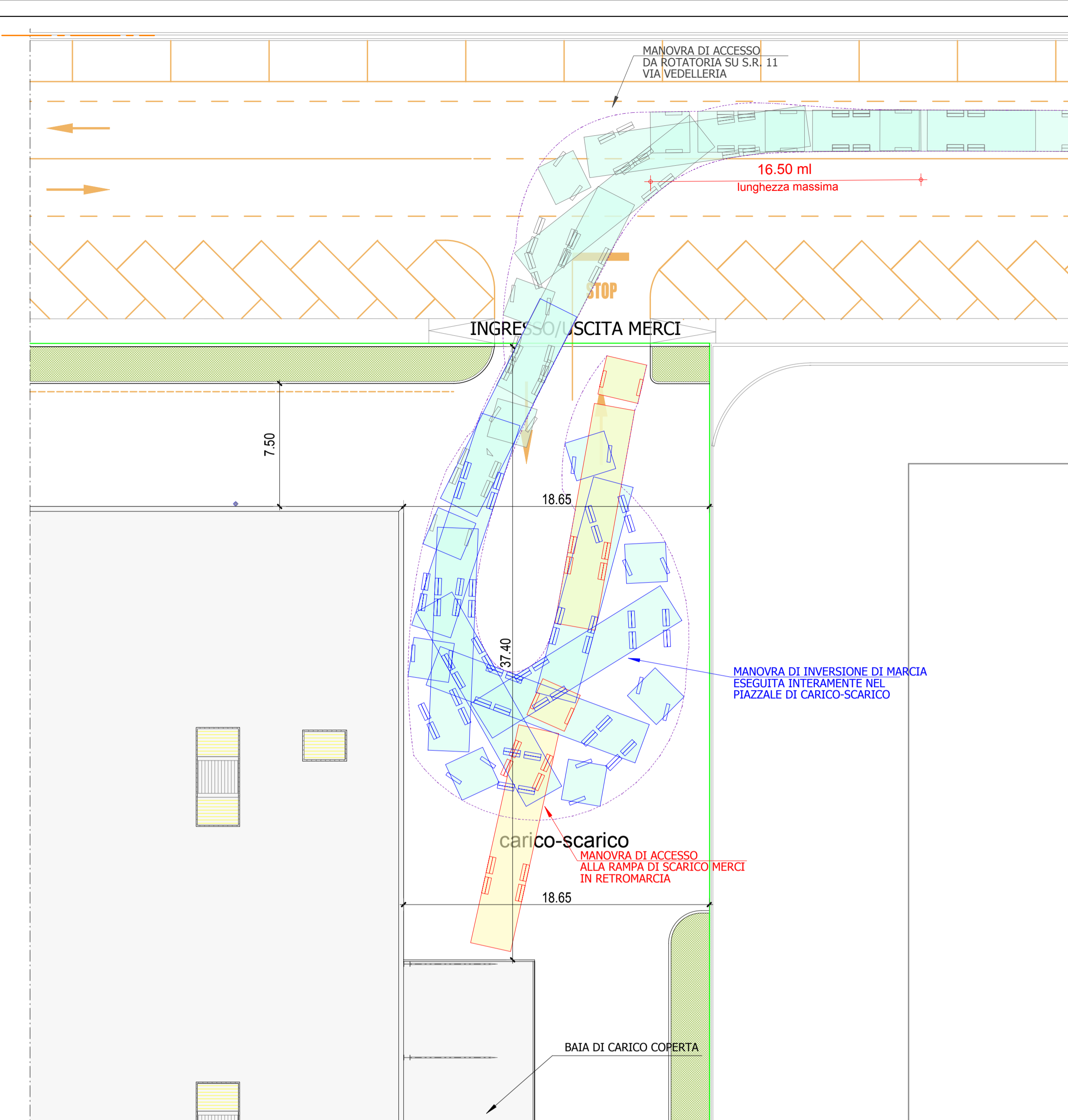
VERIFICA MANOVRE DI ACCESSO DEGLI AUTOMEZZI ALL'AREA DI CARICO-SCARICO MERCI
