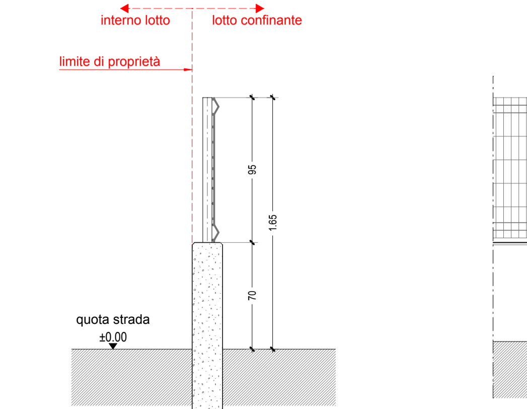
SEZ. A-A
