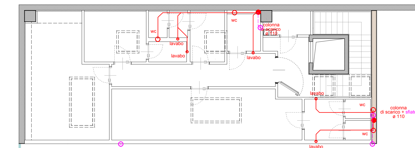
DETTAGLIO SCARICHI PIANO PRIMO - SCALA 1:100
