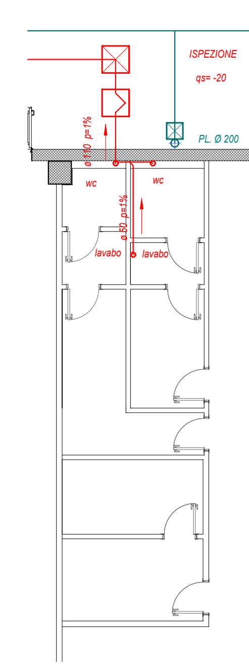
DETTAGLIO SCARICHI PIANO TERRA - SCALA 1:100
