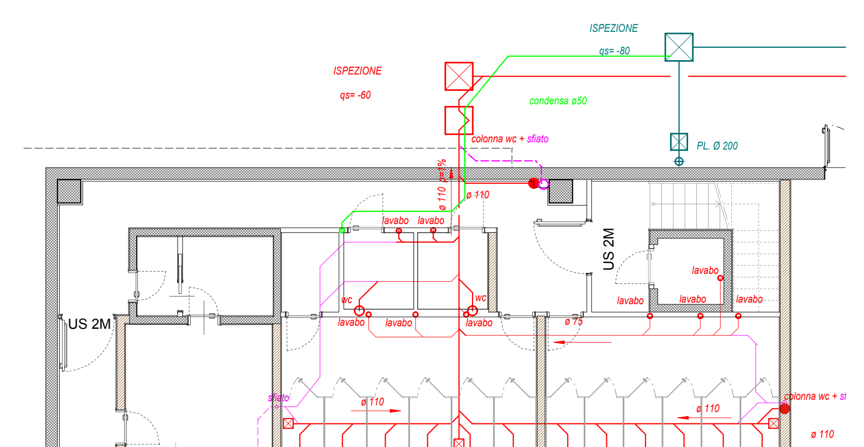
DETTAGLIO SCARICHI PIANO PRIMO - SCALA 1:100
