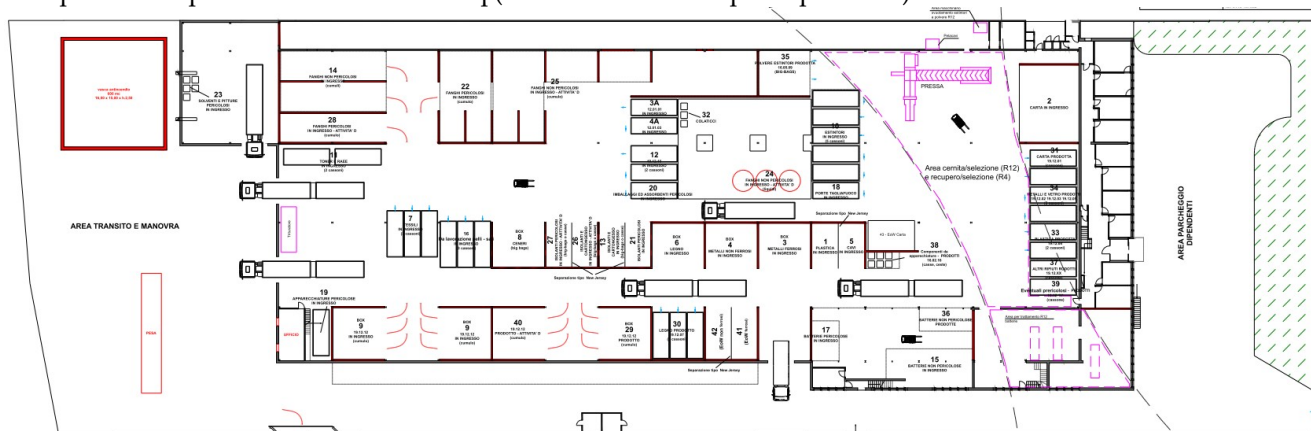
Layout dell'impianto
