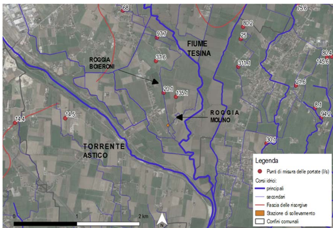
Figura 4 - Reticolo superficiale nei pressi della stazione di sollevamento
