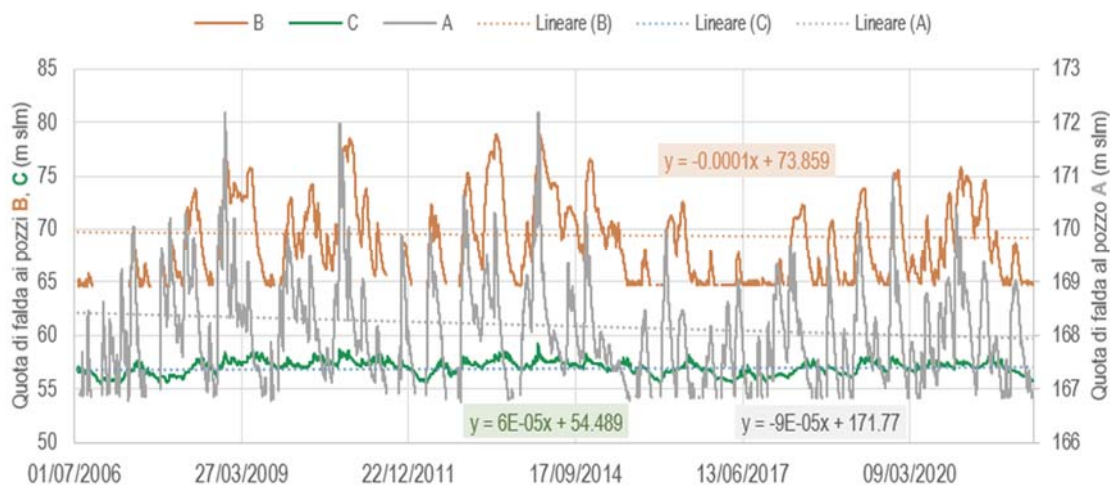
Figura 3 - Andamento della quota di falda presso le tre stazioni di monitoraggio con individuazione della retta di tendenza
