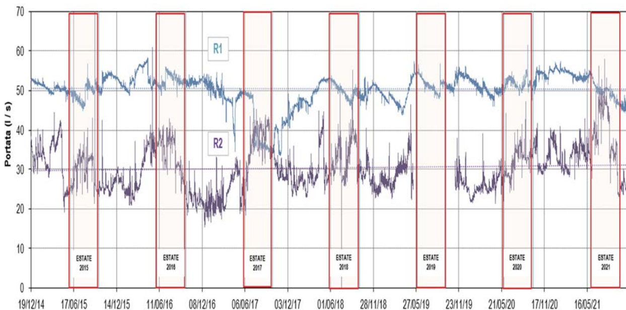
Figura 6 - Valori di portata calcolati presso le risorgive R1 e R2
