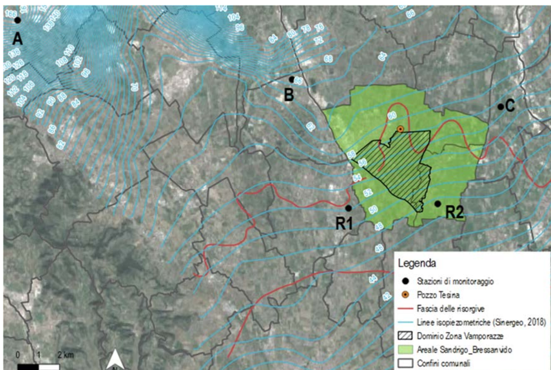
Figura 2 - Ubicazione delle stazioni di monitoraggio del regime piezometrico e di risorgiva sovrapposte al campo di flusso della falda (archivio Sinerggeo)
