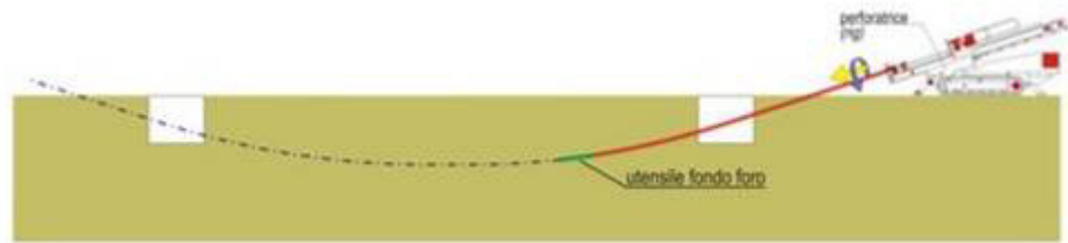
Figura 13 Perforazione pilota (pilot bore)
