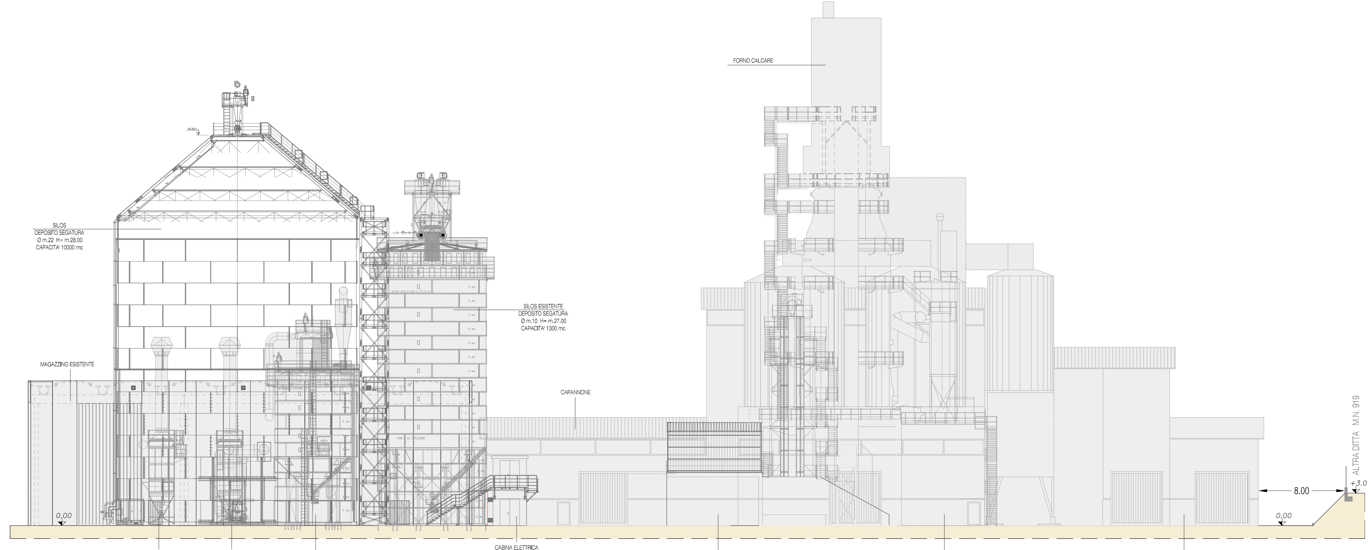
PROSPETTO NORD - EST scala 1:200
