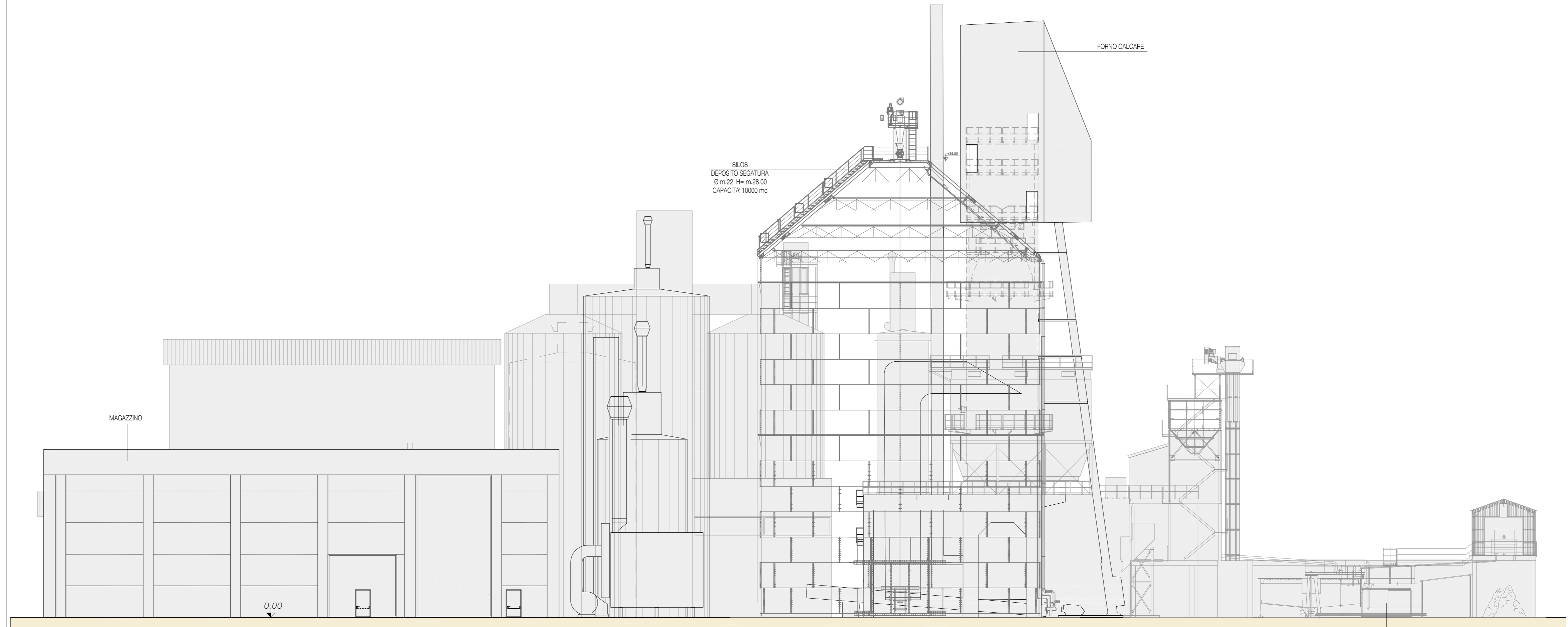
PROSPETTO SUD - EST scala 1:200
