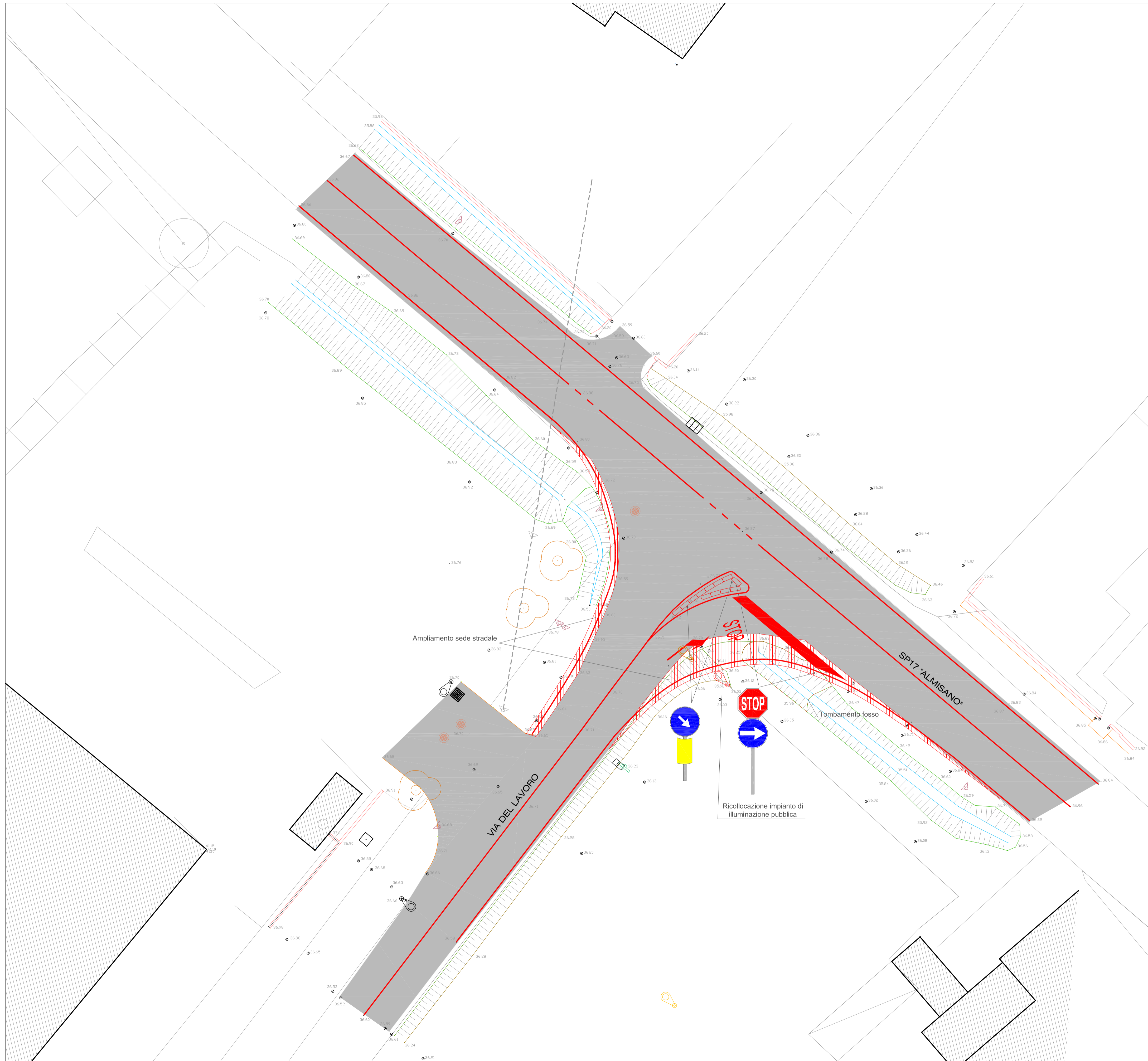
STATO COMPARATO - Scala 1:500
