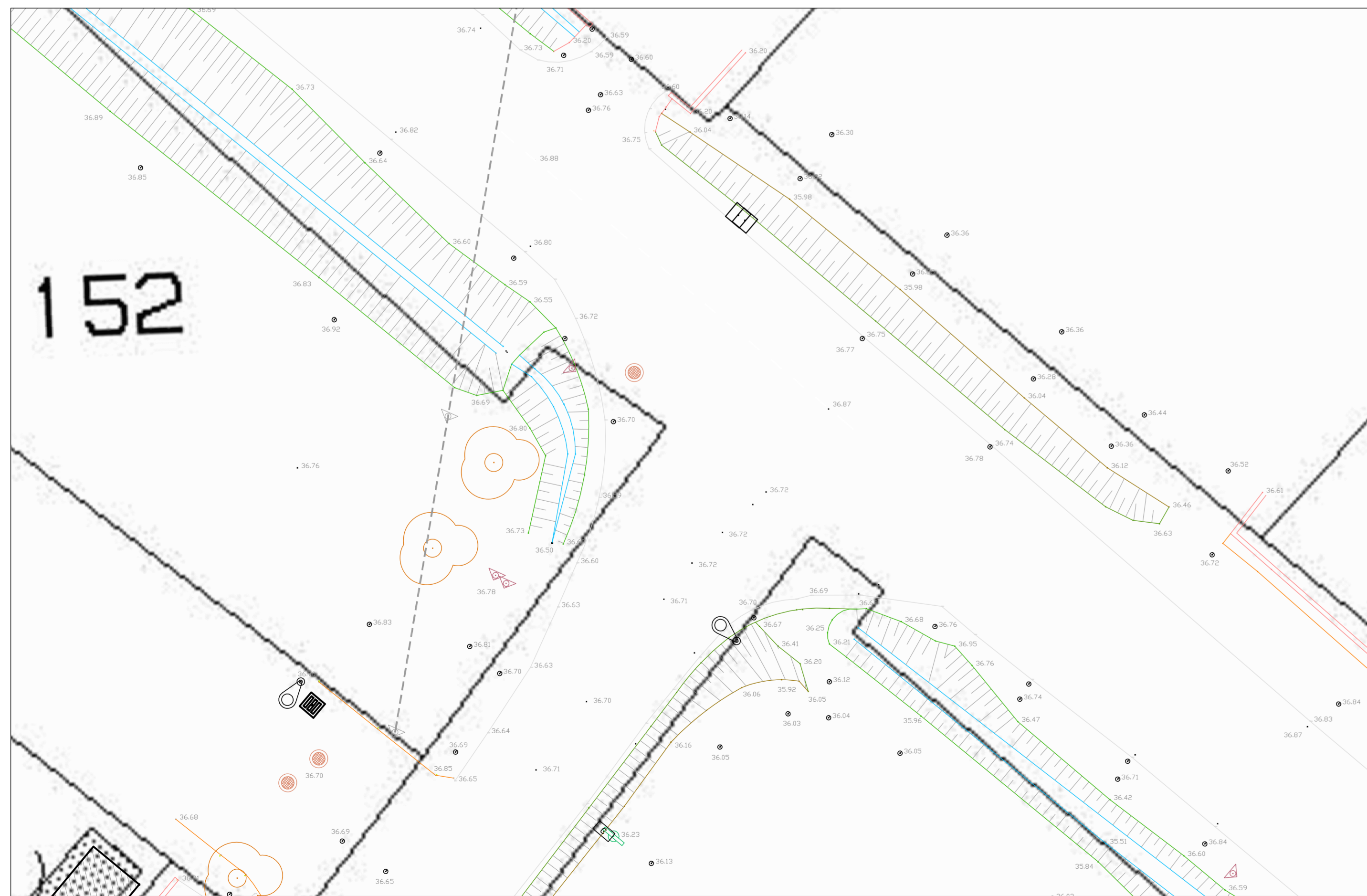
SOVRAPPOSIZIONE RILIEVO CON ESTRATTI DI MAPPA CATASTALE - Scala 1: 500
