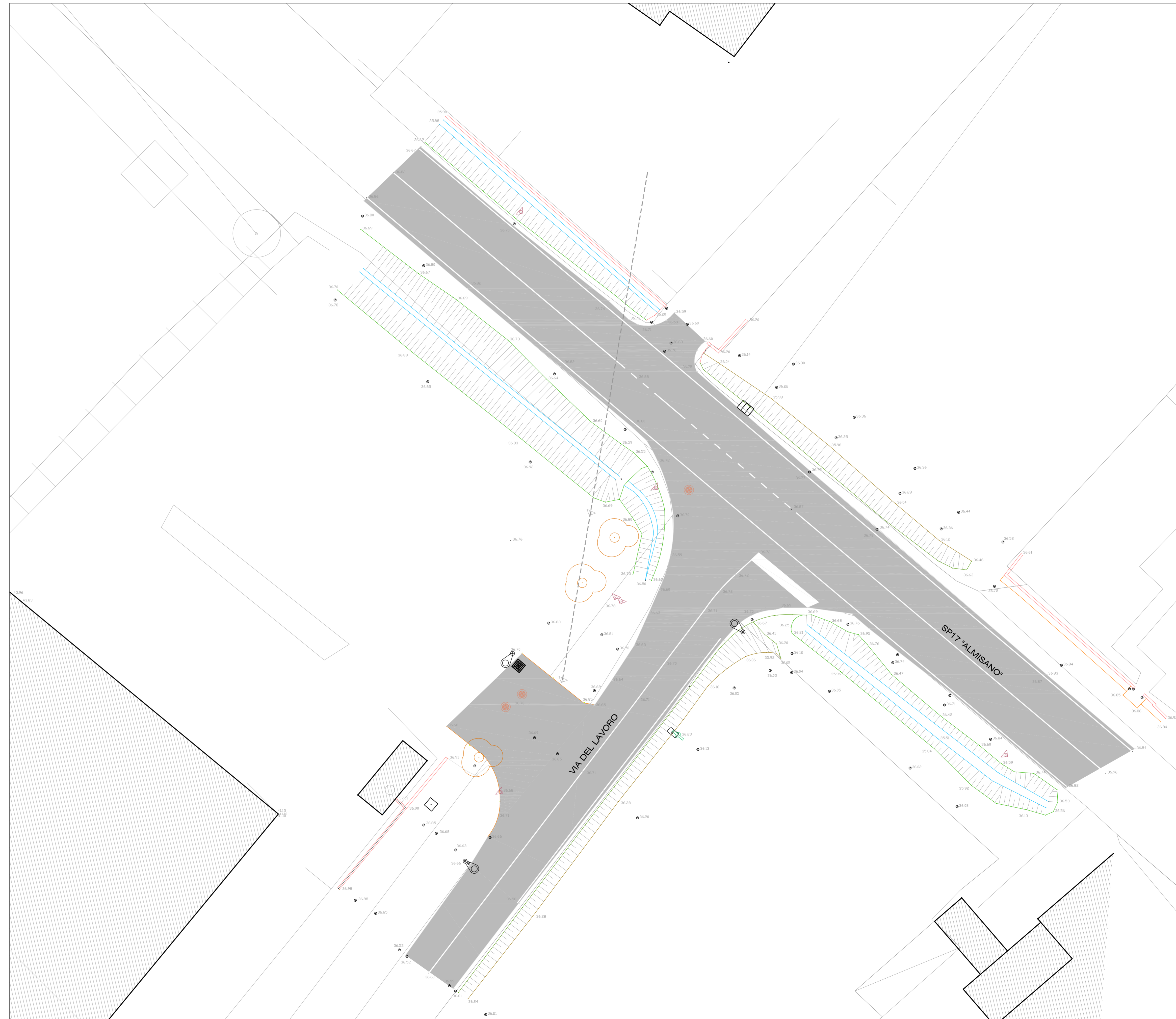
RILIEVO STATO DI FATTO - Scala 1500
