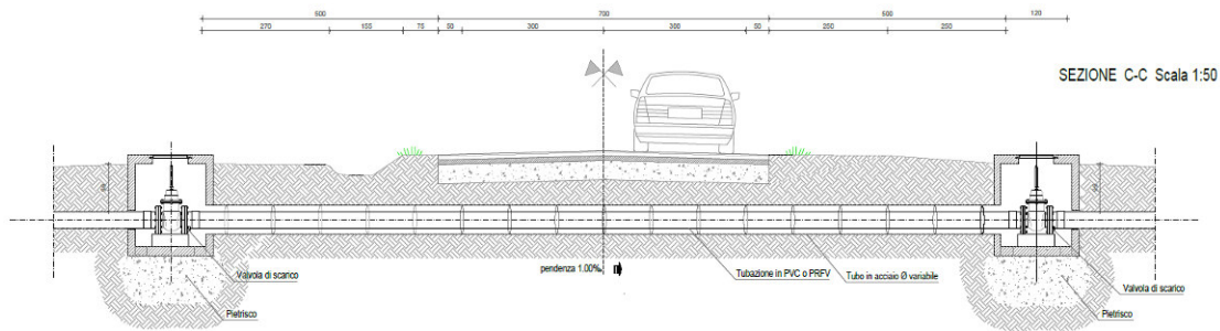
Figura 4 sezione tipo di attraversamento stradale.
