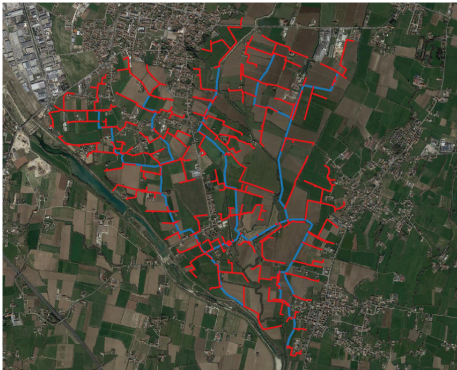
Figura 3 rete di progetto, in blu il sistema principale e rosso il secondario.
