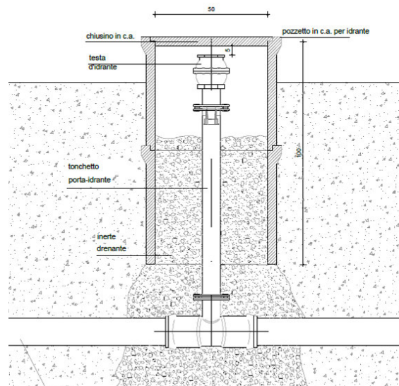
Figura 7 sezione tipo degli idranti.
