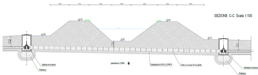
Figura 5 sezione attraversamento del Tesina.
