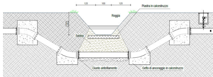
Figura 6 sezione tipo attraversamento rogge e canali.
