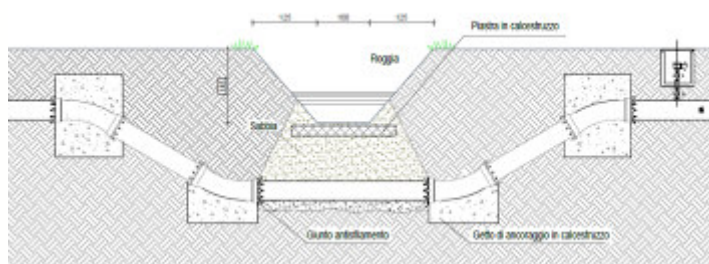
Figura 32 sezione tipo attraversamento rogge e canali.
