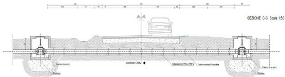
Figura 30 sezione tipo di attraversamento stradale.
