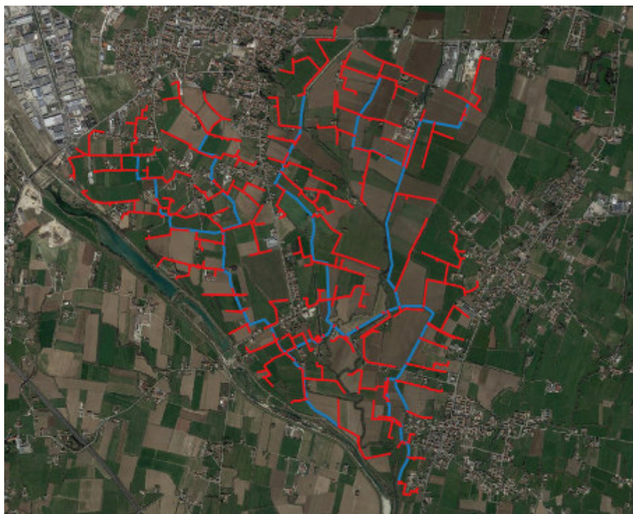
Figura 29 rete di progetto, in blu il sistema principale e rosso il secondario.
