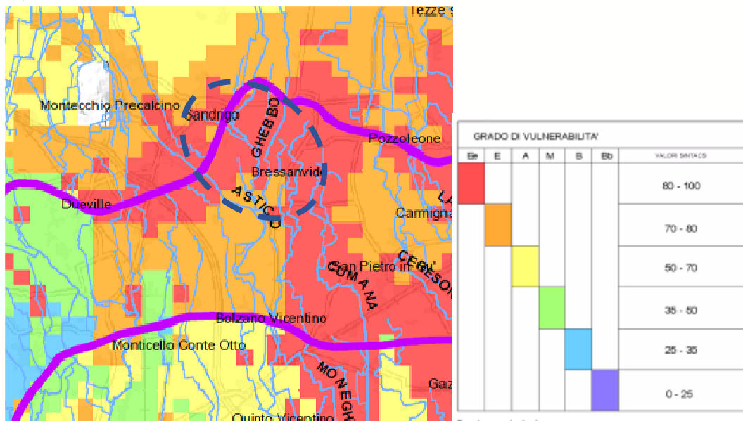
Figura 11 Estratto della Carta della Vulnerabilità Intrinseca di Falda.
