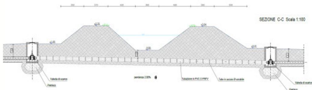
Figura 31 sezione attraversamento del Tesina.
