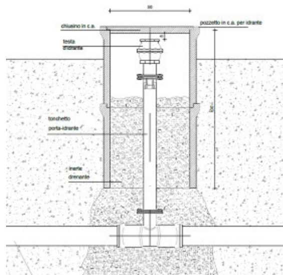
Figura 33 sezione tipo degli idranti.
