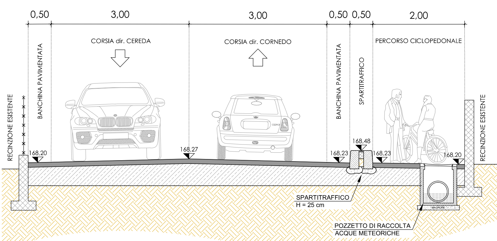
SEZIONE 2 - progetto
