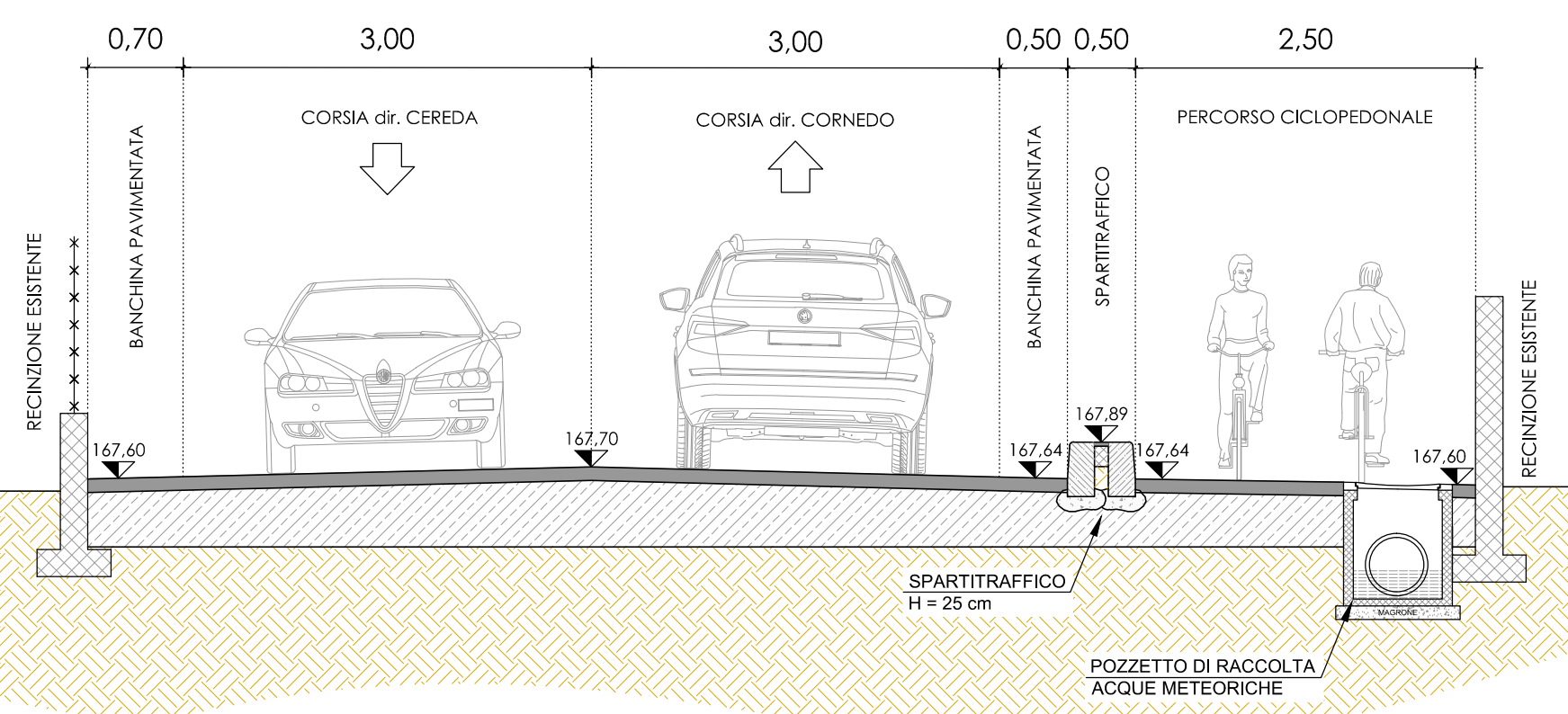
SEZIONE 1 - progetto
