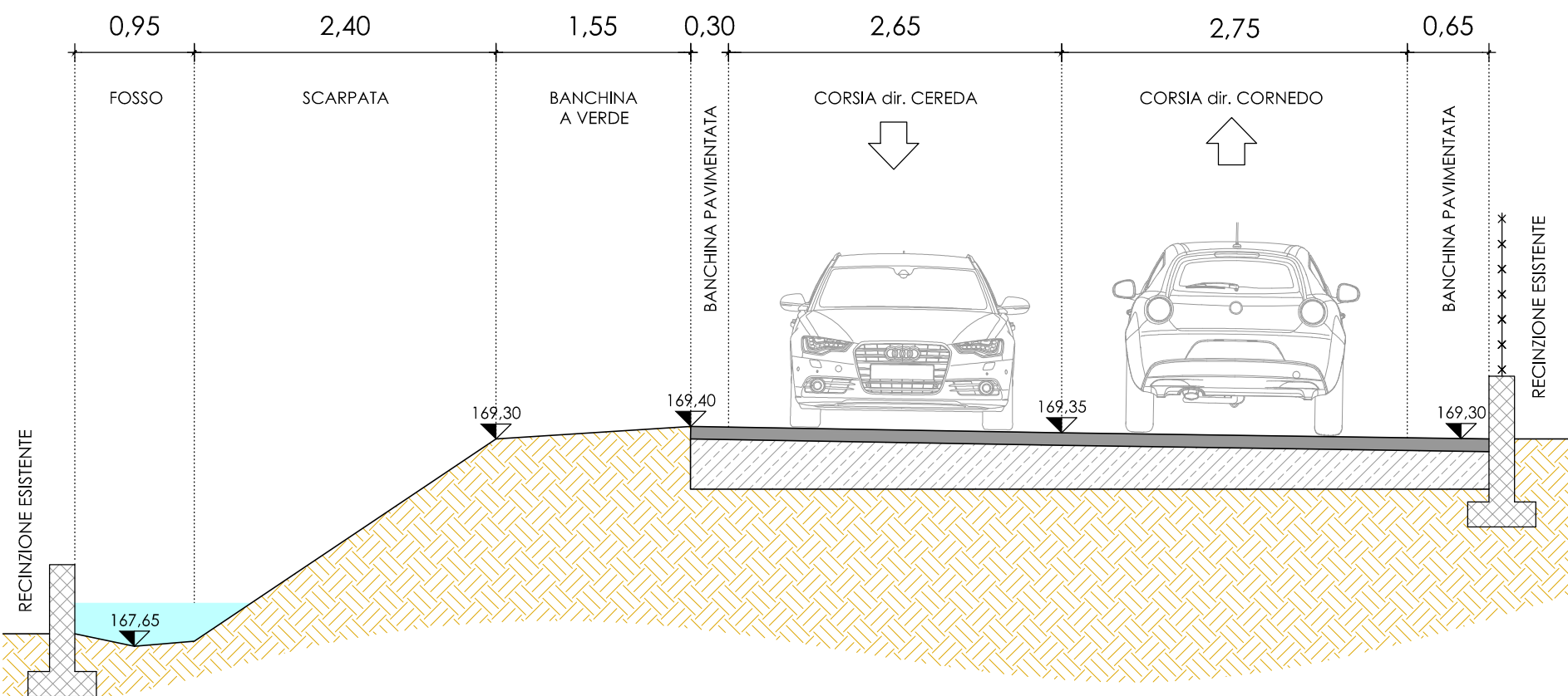
SEZIONE 3 - progetto
