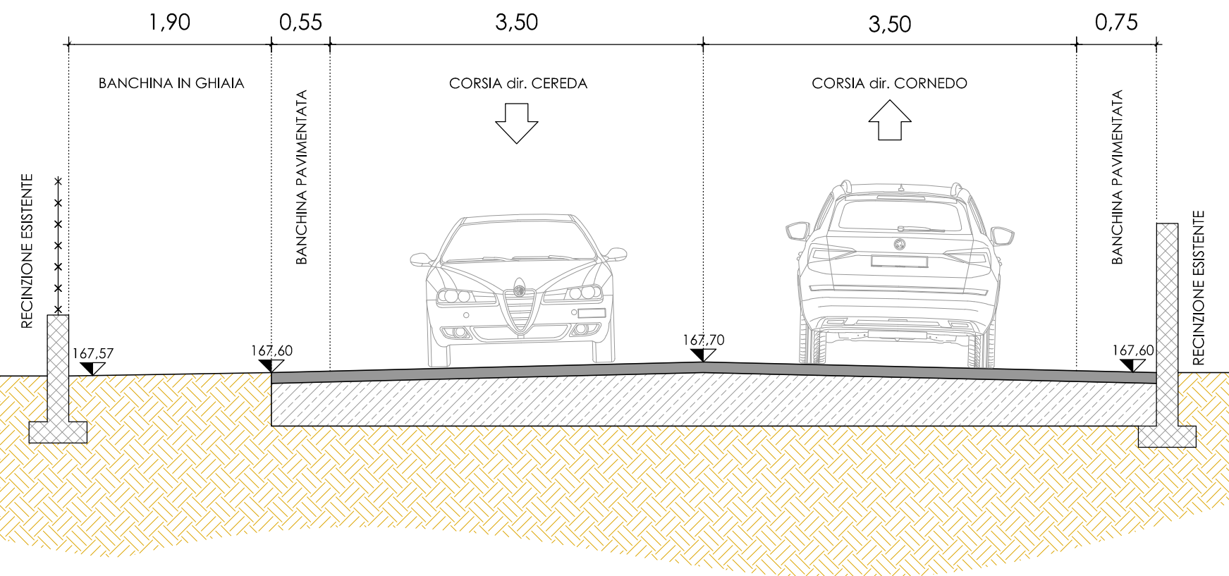
SEZIONE 1 - progetto
