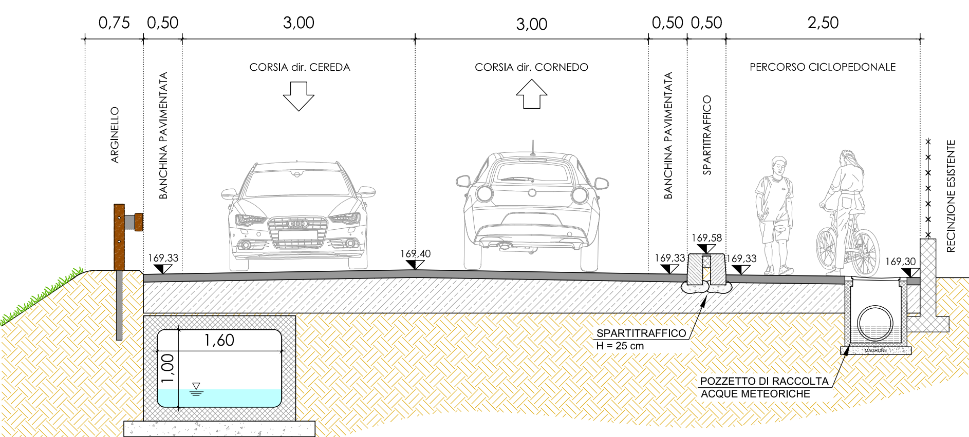
SEZIONE 3 - progetto
