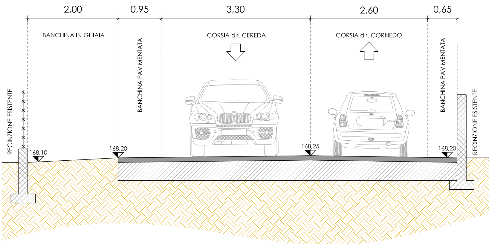
SEZIONE 2 - progetto
