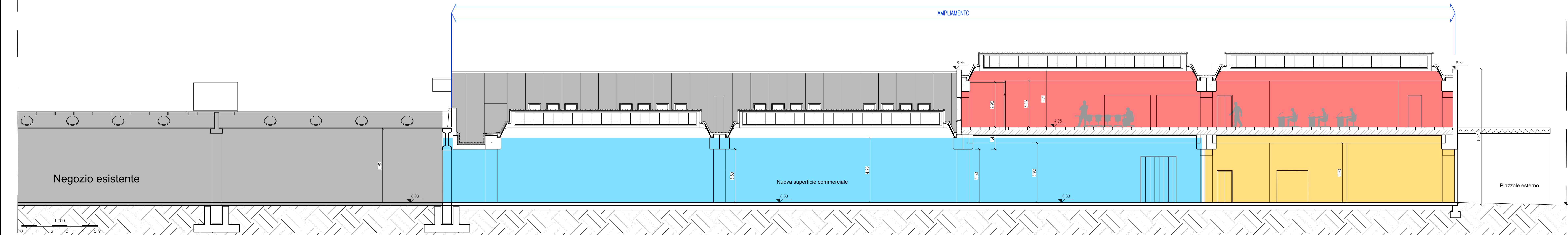
SEZIONE C-C
