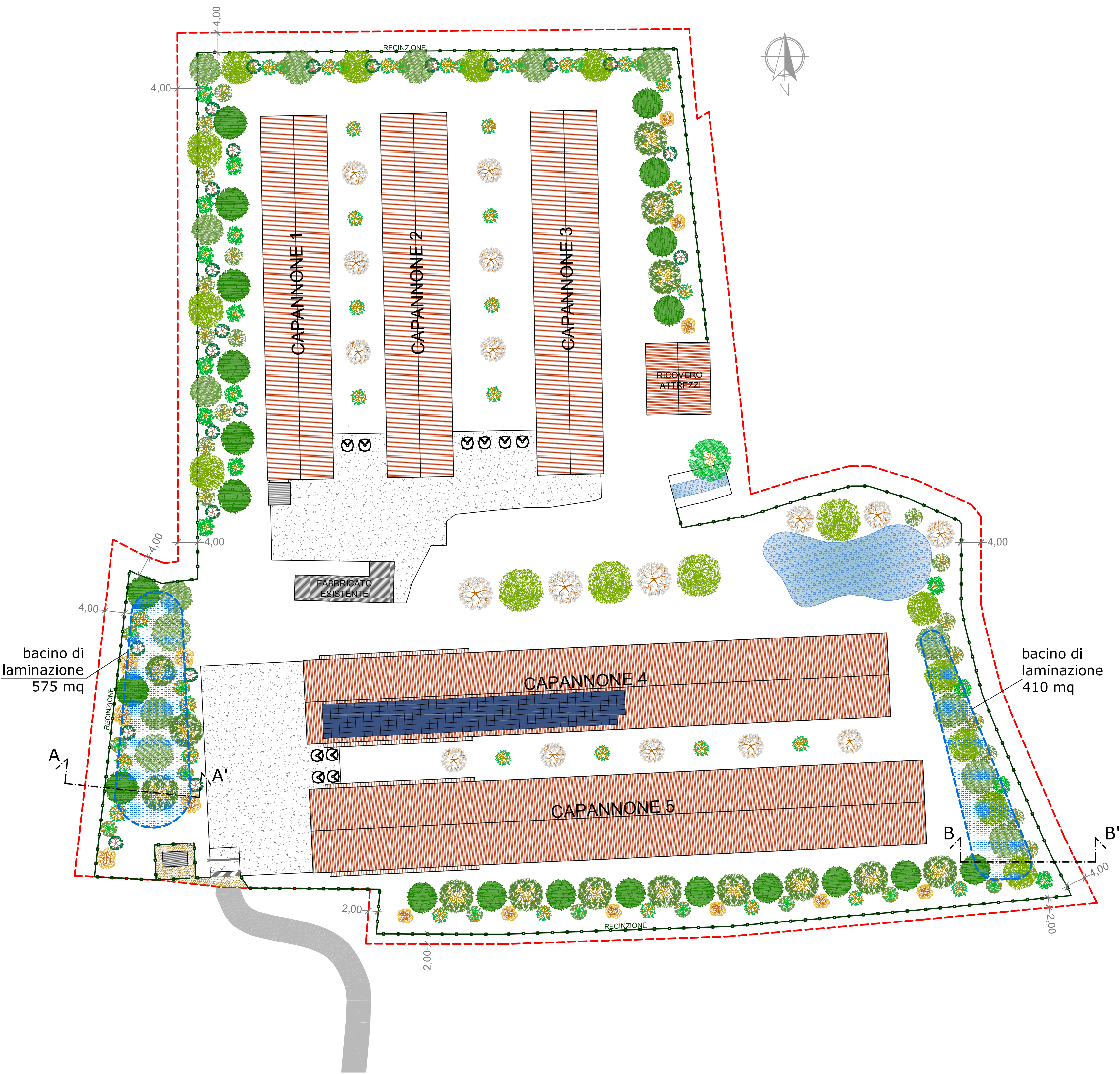
PLANIMETRIA GENERALE - scala 1:500
