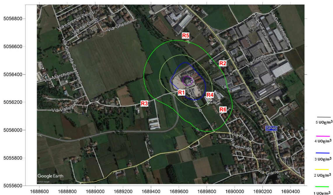
Figura 7 - Risultati della modellizzazione diffusionale. Verifica dei valori di accettabilità delle linee guida della Regione del Veneto
