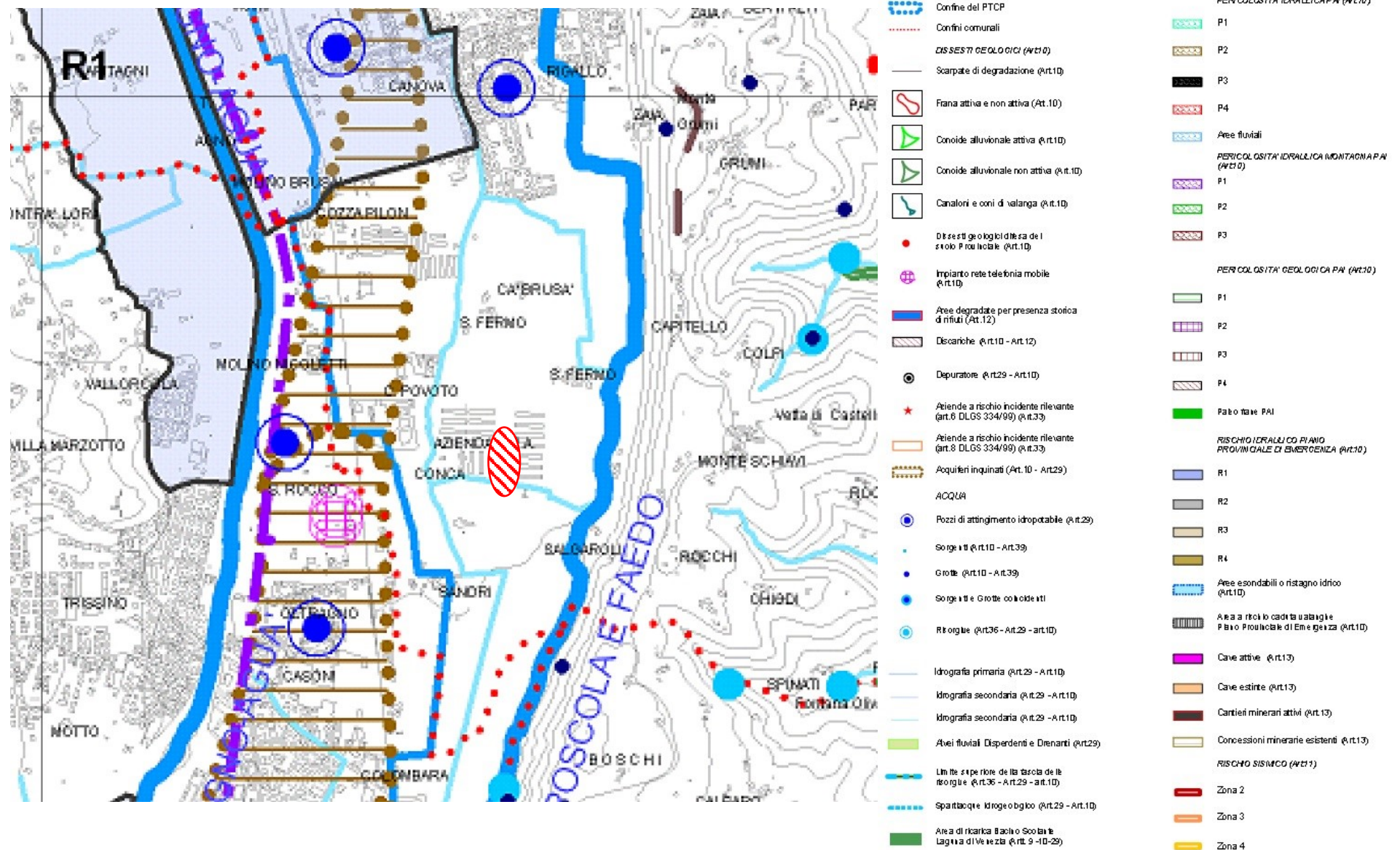
Figura 4: Estratto della Tavola 2.1.B - Carta della Fragilità.
