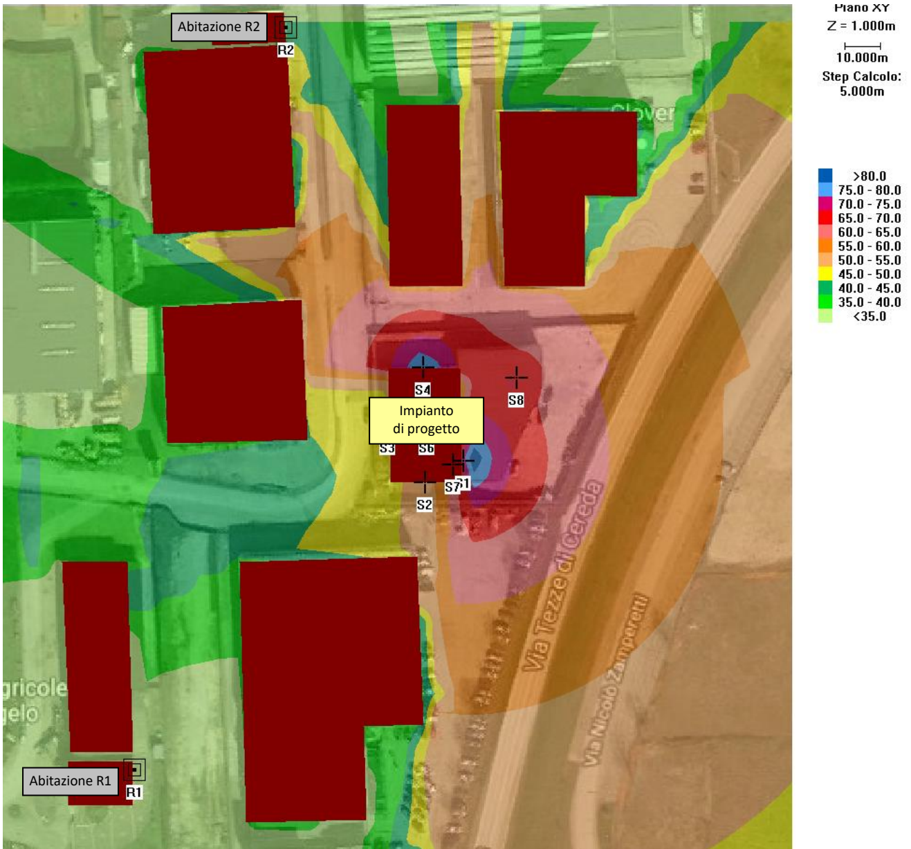
FIGURA 27: MODELLO DI PROPAGAZIONE DELLE ISOFONE – STATO PREVISIONALE (VALORI IN DB).
