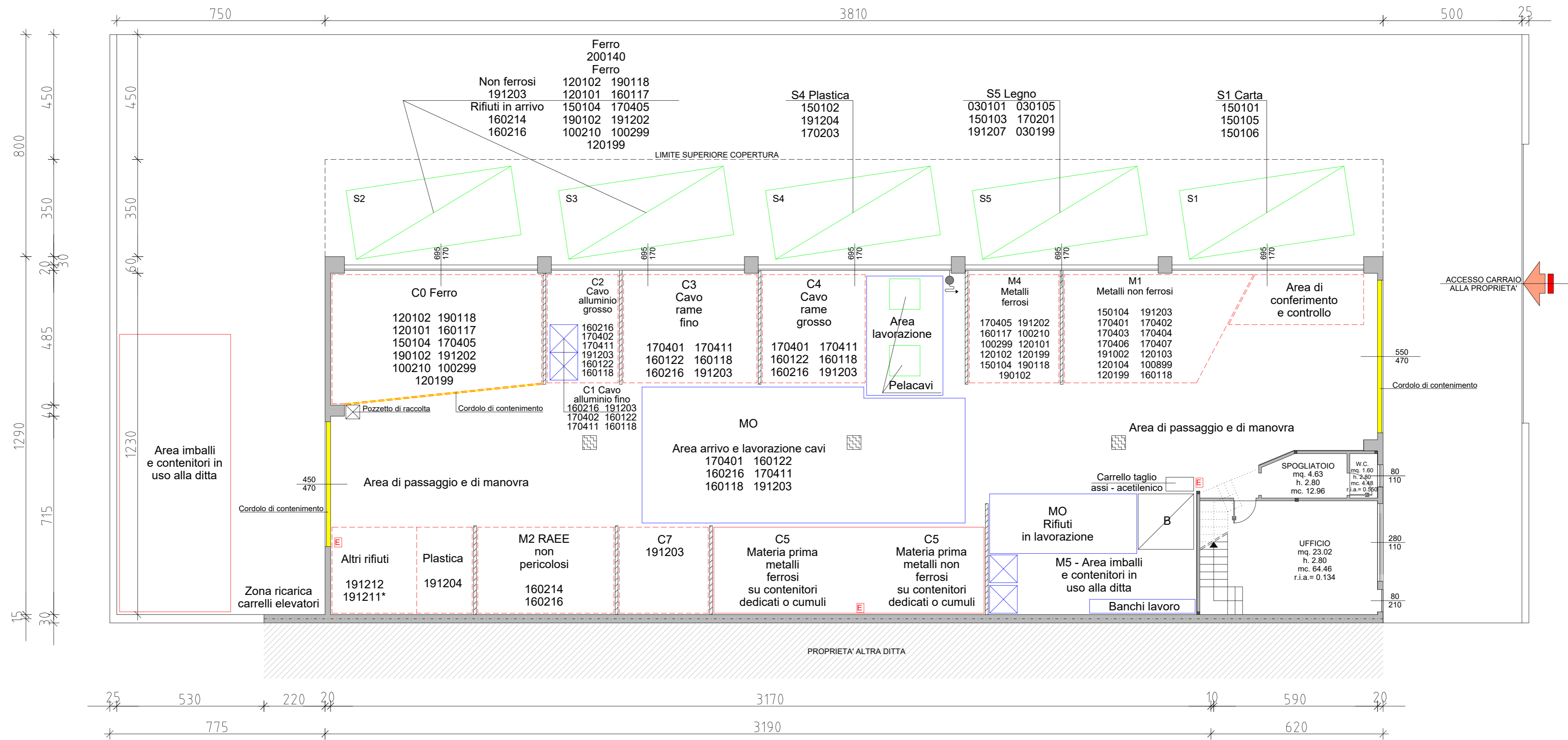
PIANTA PIANO TERRA * Lay - Out Distributivo * scala 1:100
