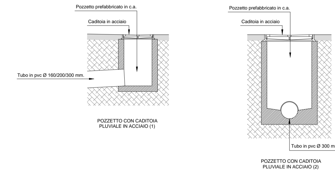
POZZETTO CON CADITOIA PLUVIALE IN ACCIAIO (2)
