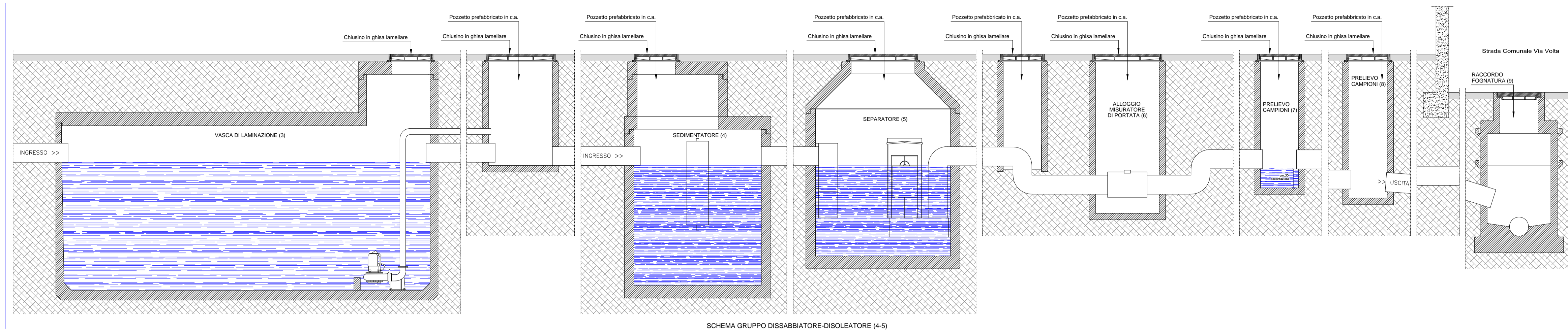
SCHEMA GRUPPO DISSABBIATORE-DISOLEATORE (4-5)
