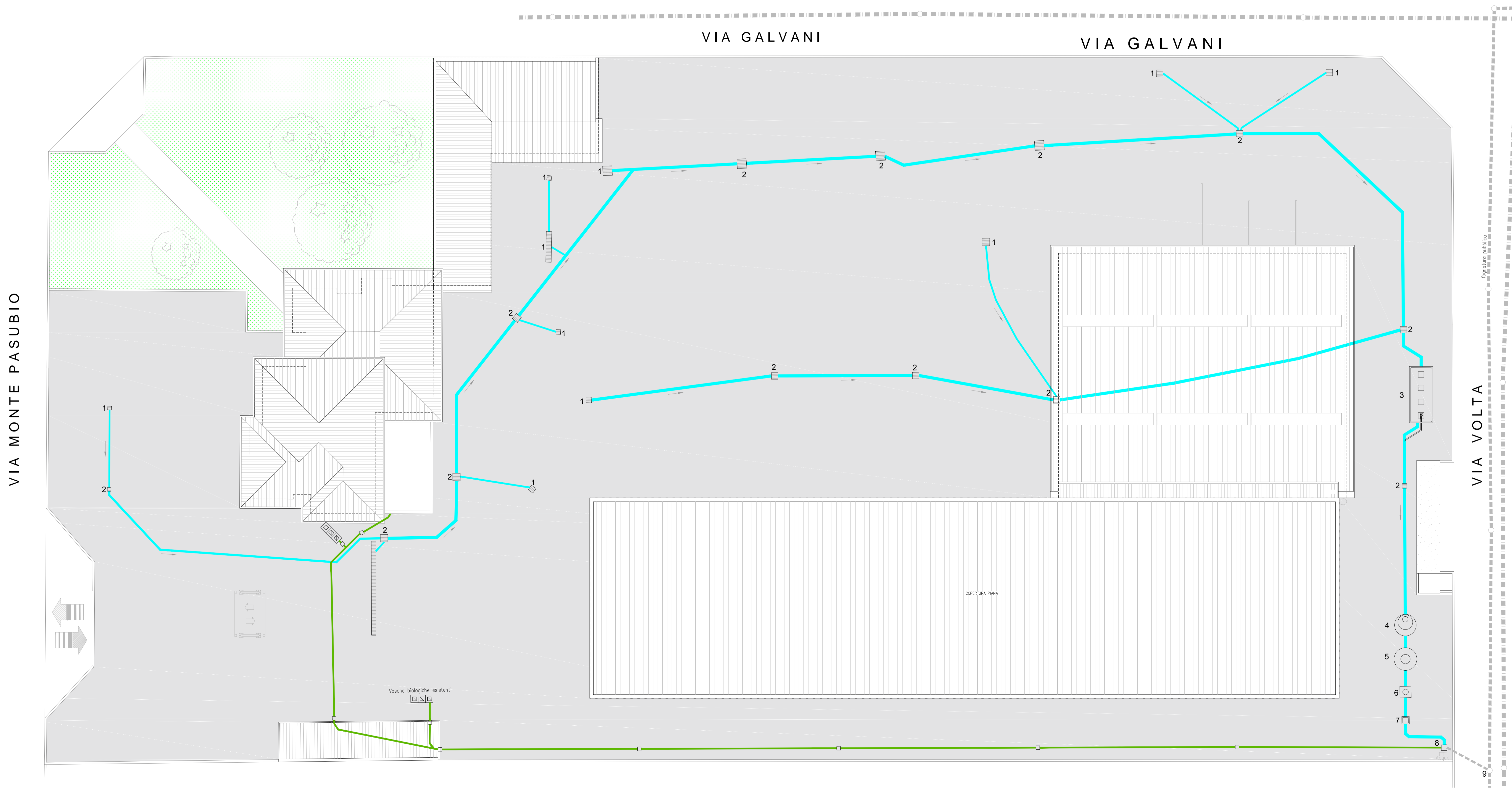
SCHEMA GRUPPO DISSABBIATORE-DISOLEATORE (4-5)
