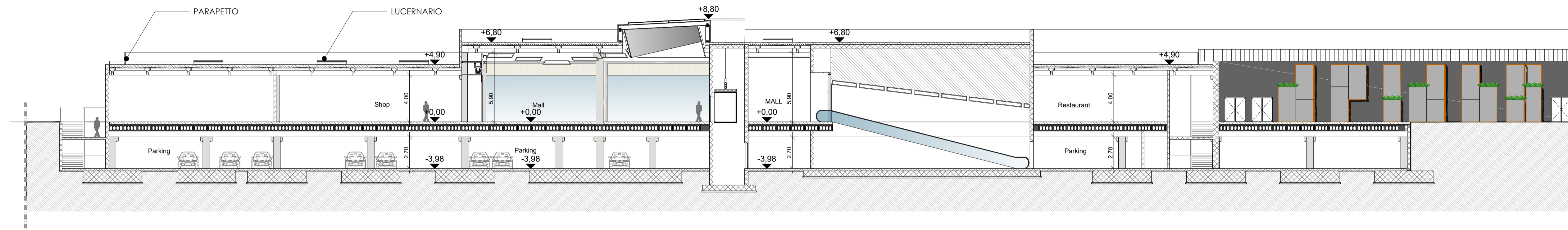
SEZIONE EE scala 1:200
