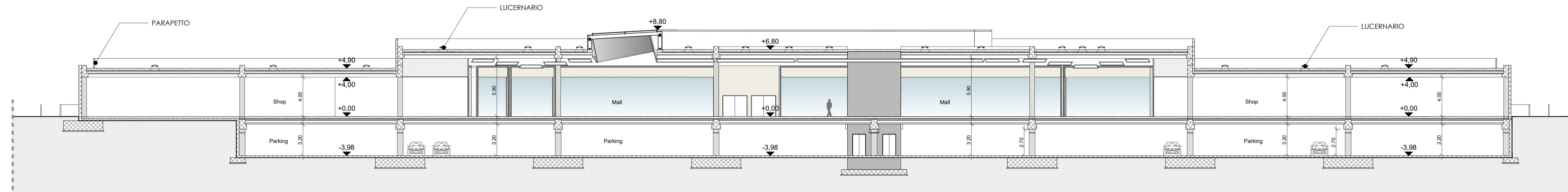
SEZIONE FF scala 1:200
