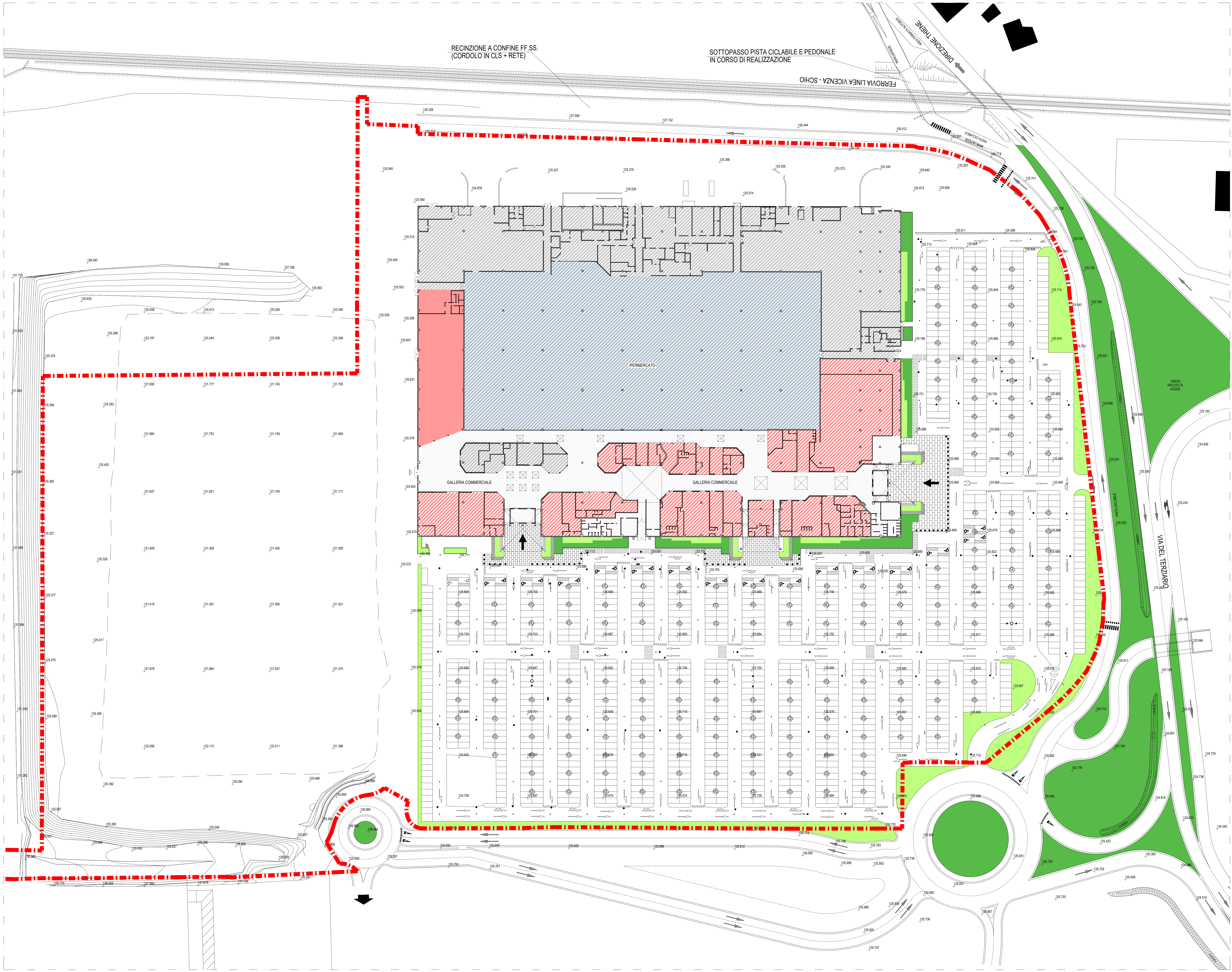
PLANIMETRIA STATO DI FATTO
