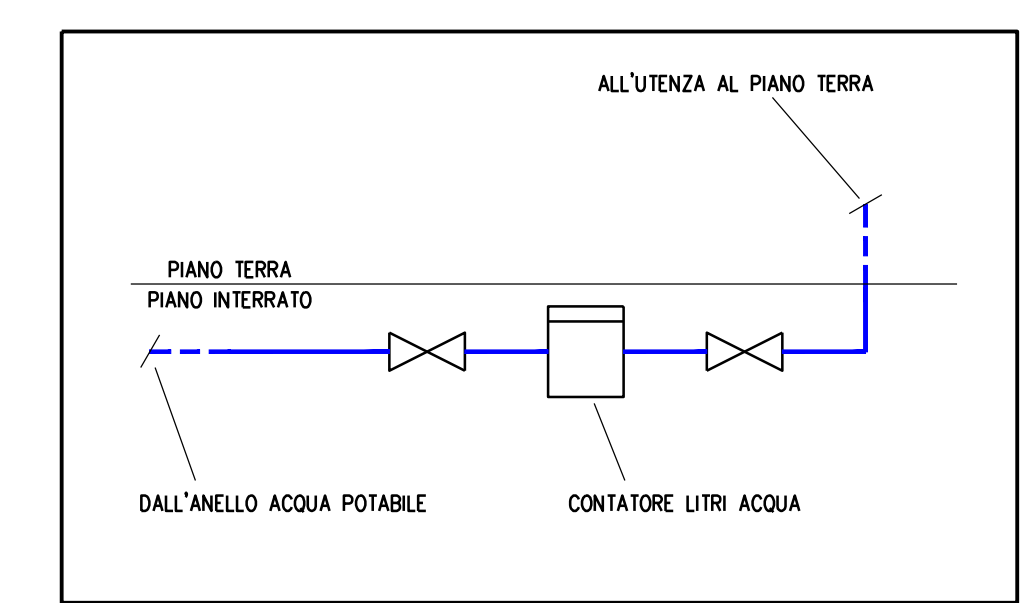
TIPICO STACCHI COLLEGAMENTO UTENZE ACQUA POTABILE
