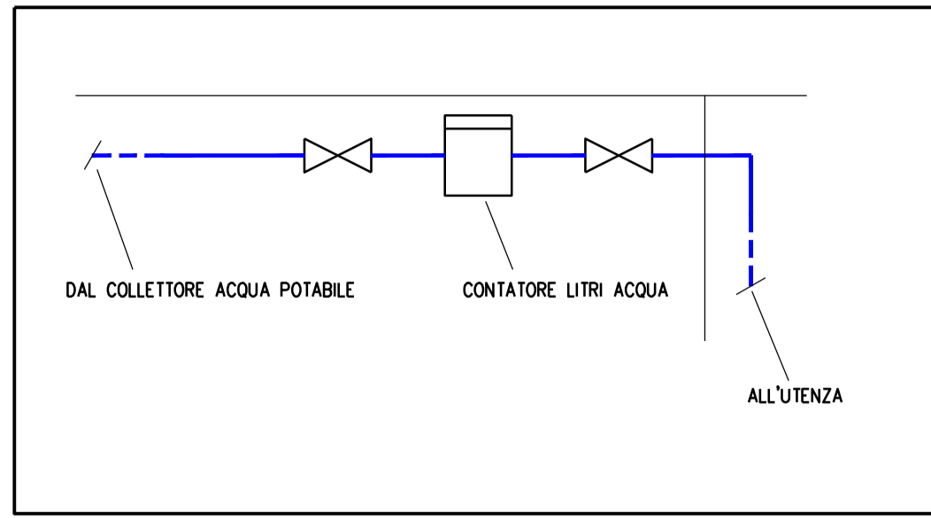
TIPICO STACCHI COLLEGAMENTO UTENZE ACQUA POTABILE
