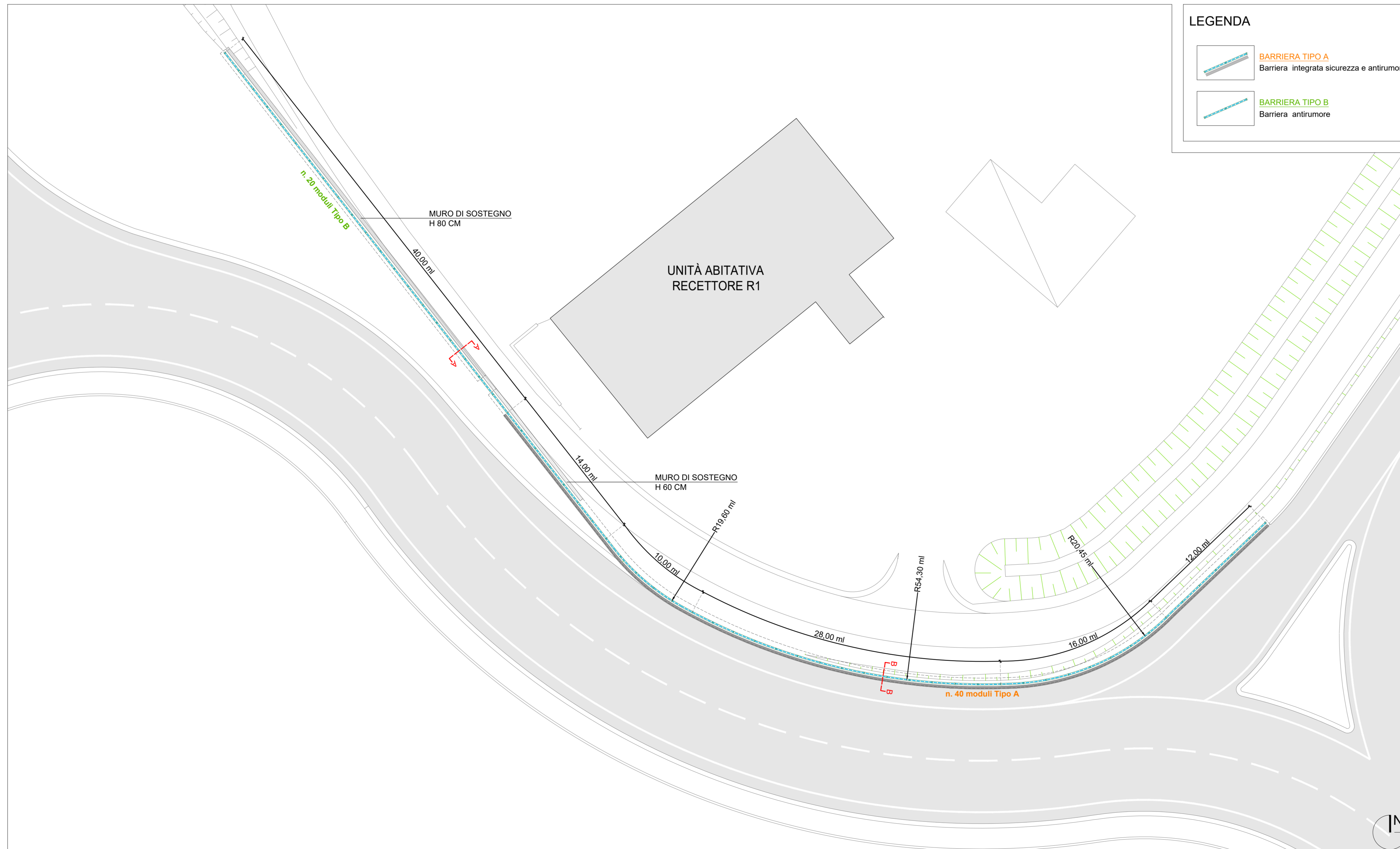
PIANTA BARRIERA INTEGRATA Scala 1:200
