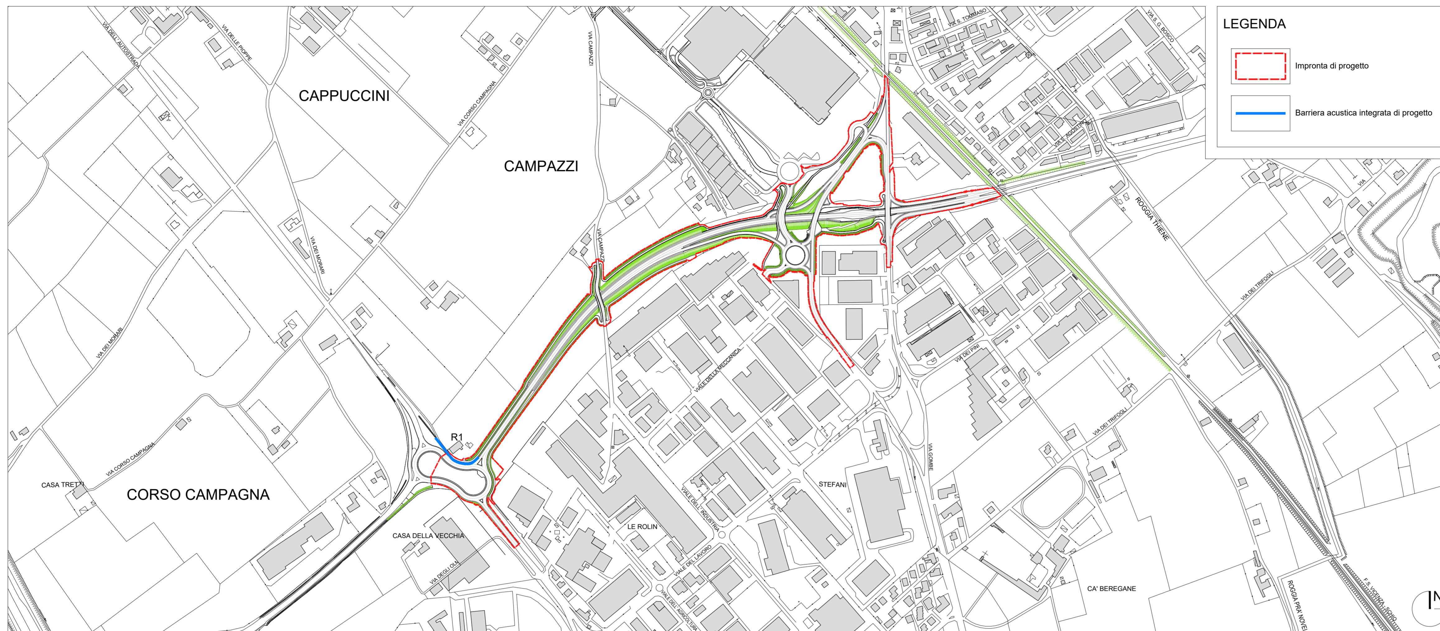
PLANIMETRIA GENERALE CON INDIVIDUAZIONE BARRIERA ACUSTICA INTEGRATA Scala 1:1.000
