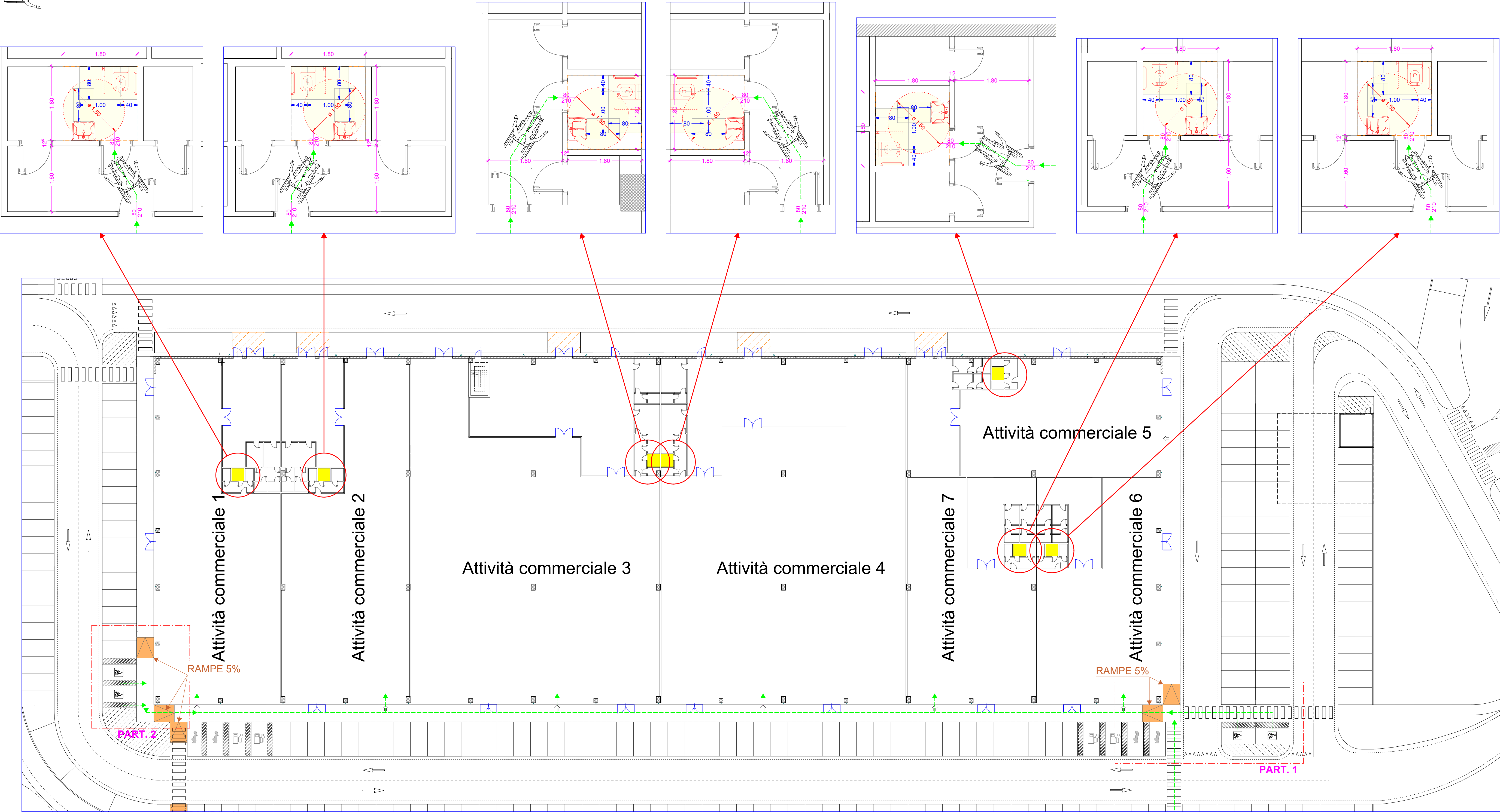
PLANIMETRIA scala 1:300
