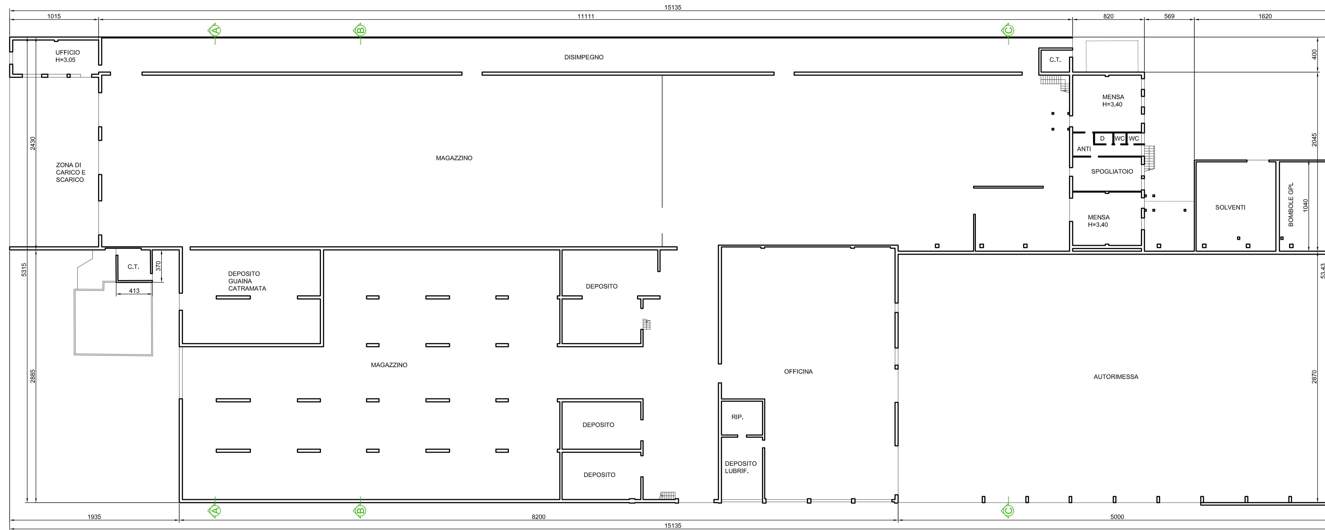
Pianta piano primo 1:250
