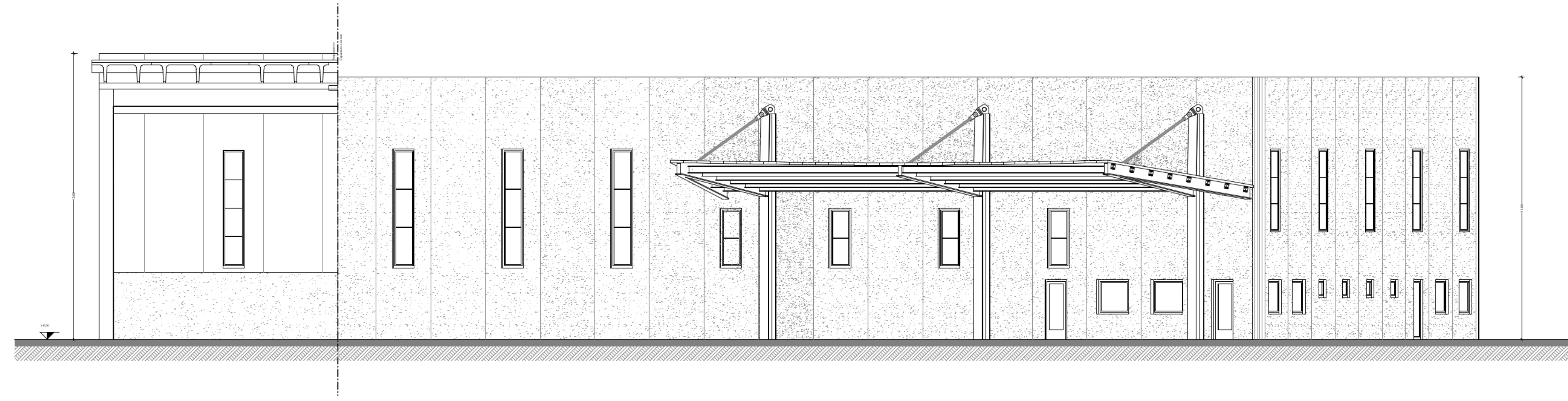
Prospetto Nord
