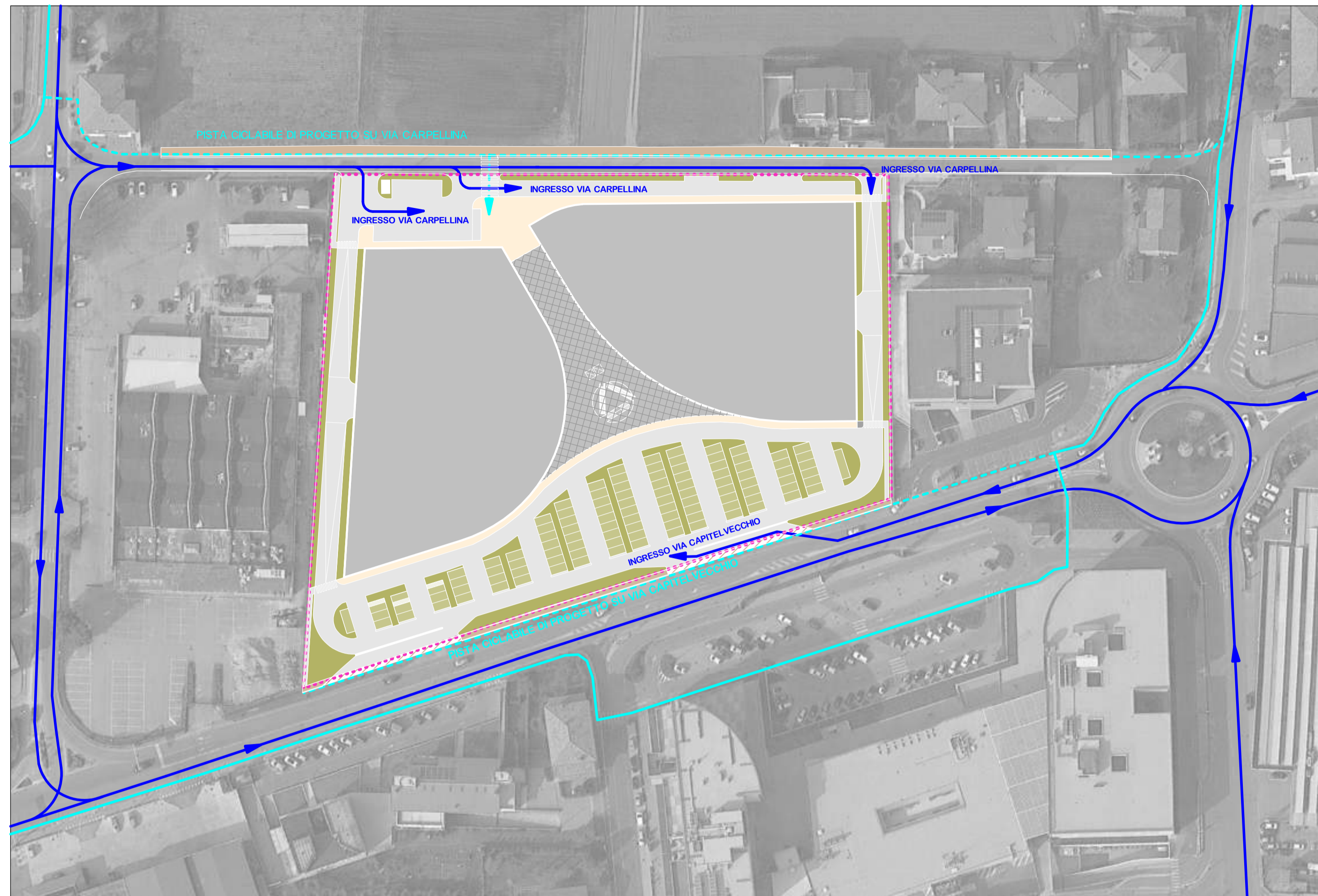
PLANIMETRIA CON INDICAZIONI VIABILITA' IN INGRESSO - SCALA 1:1000
