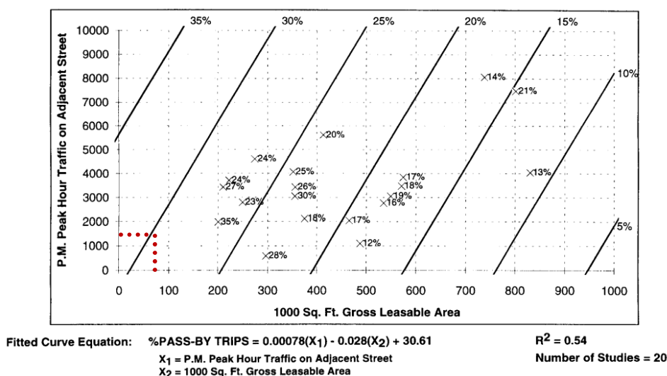
Figura 6.5 – Grafico di Peyrebrune
