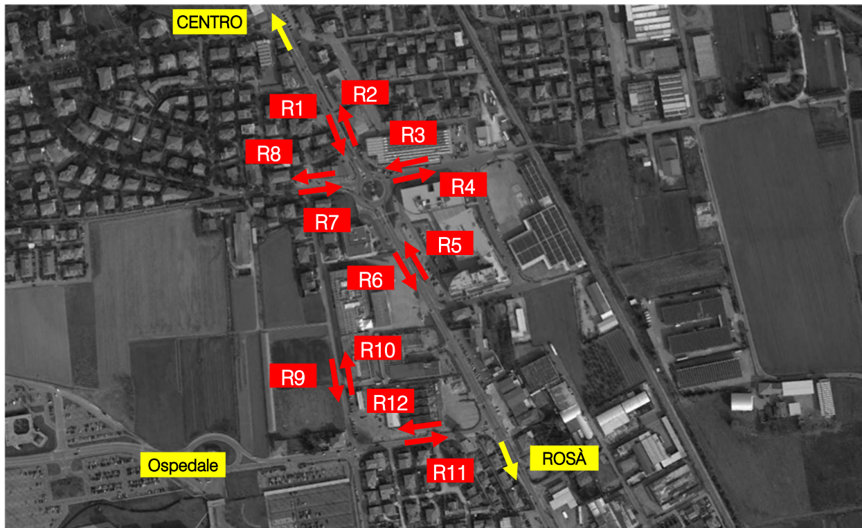
Figura 5.3 – Sezioni di rilievo tramite strumentazione radar
