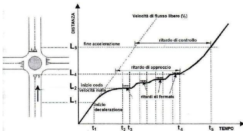
Figura 8.2 – Definizione tipologie di ritardo per una rotatoria
