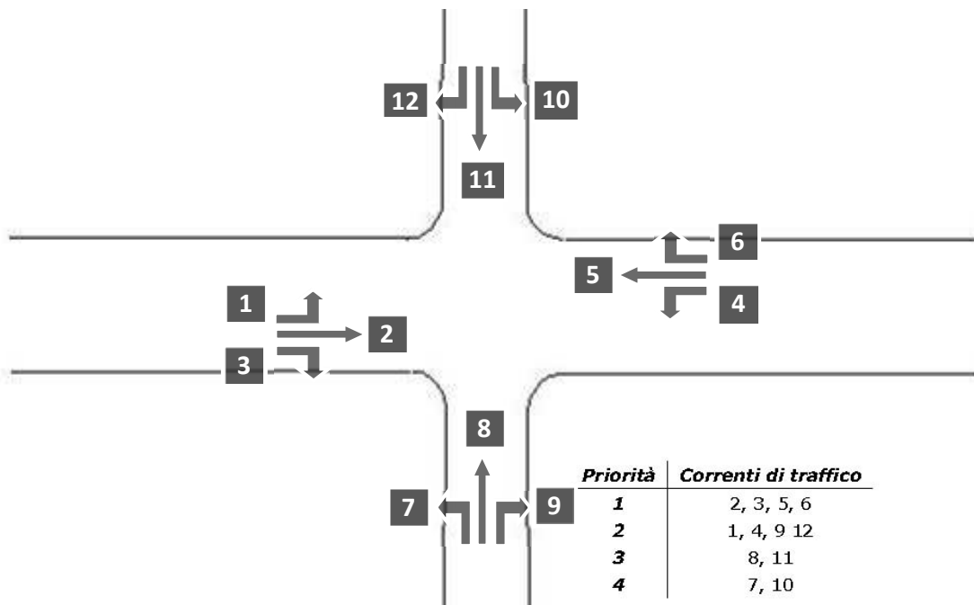
Figura 8.1 – Gerarchia delle correnti di traffico
