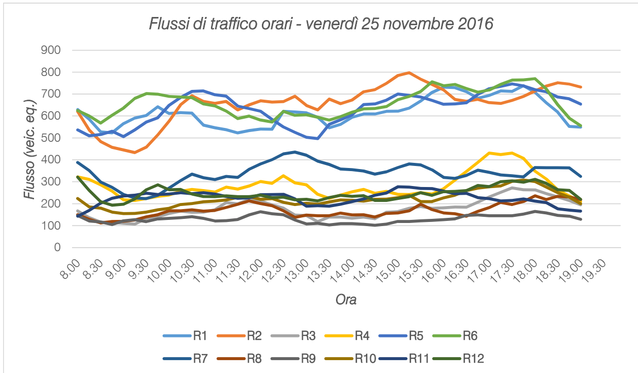
Figura 5.11 – Andamento volumi di traffico per sezione – venerdì 25.11.2016
