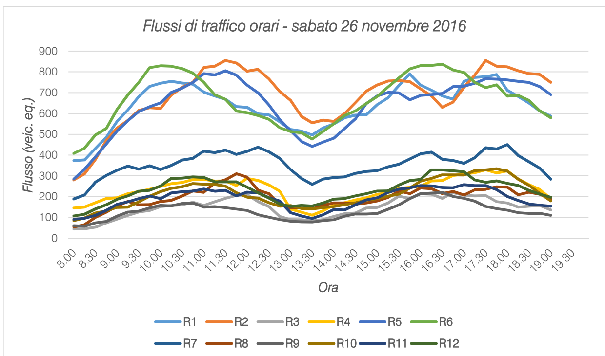
Figura 5.12 – Andamento volumi di traffico per sezione – sabato 26.11.2016
