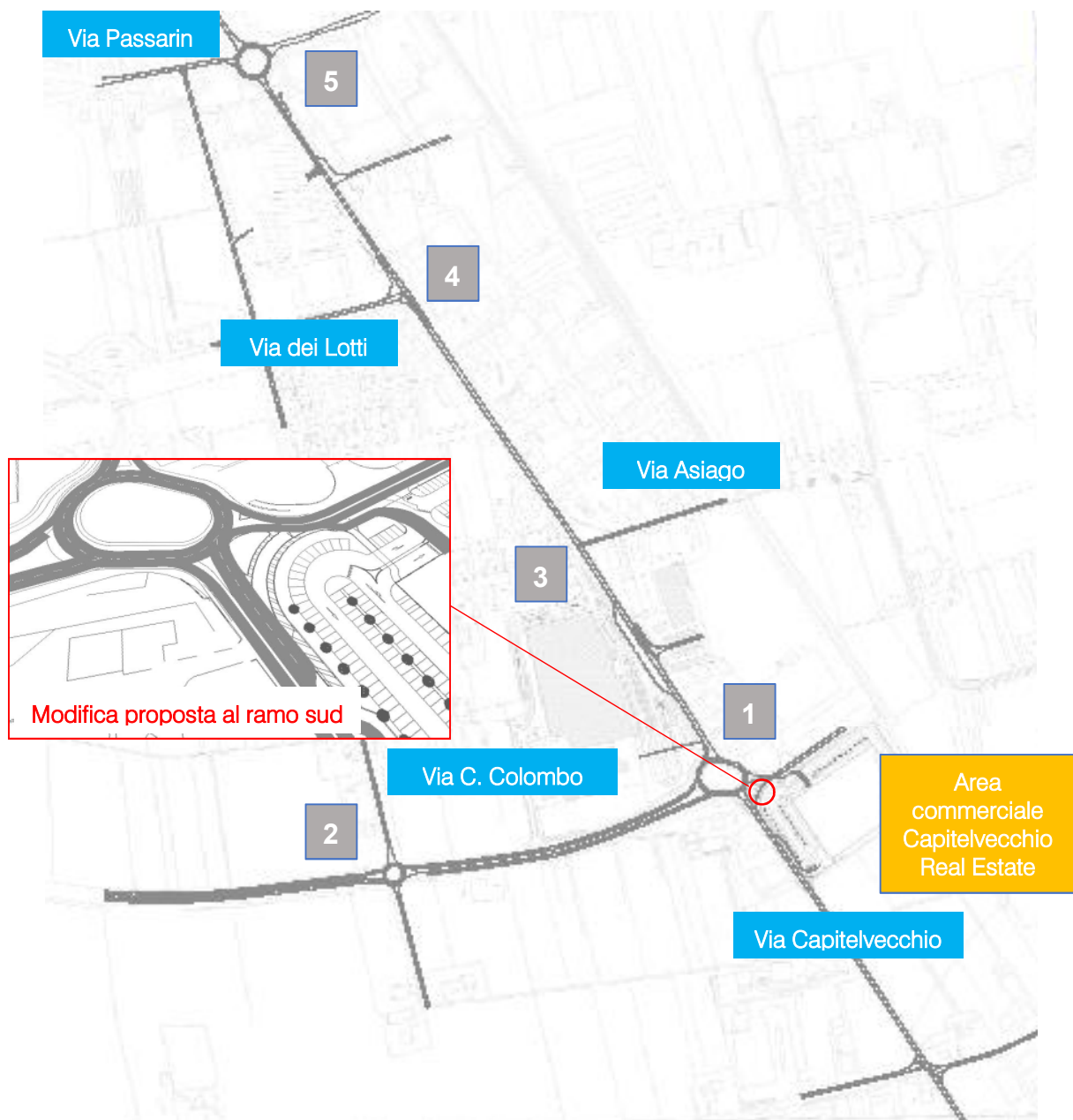
Figura 9.1 – Rete microsimulata e nodi valutati, Scenari 0 e 1
