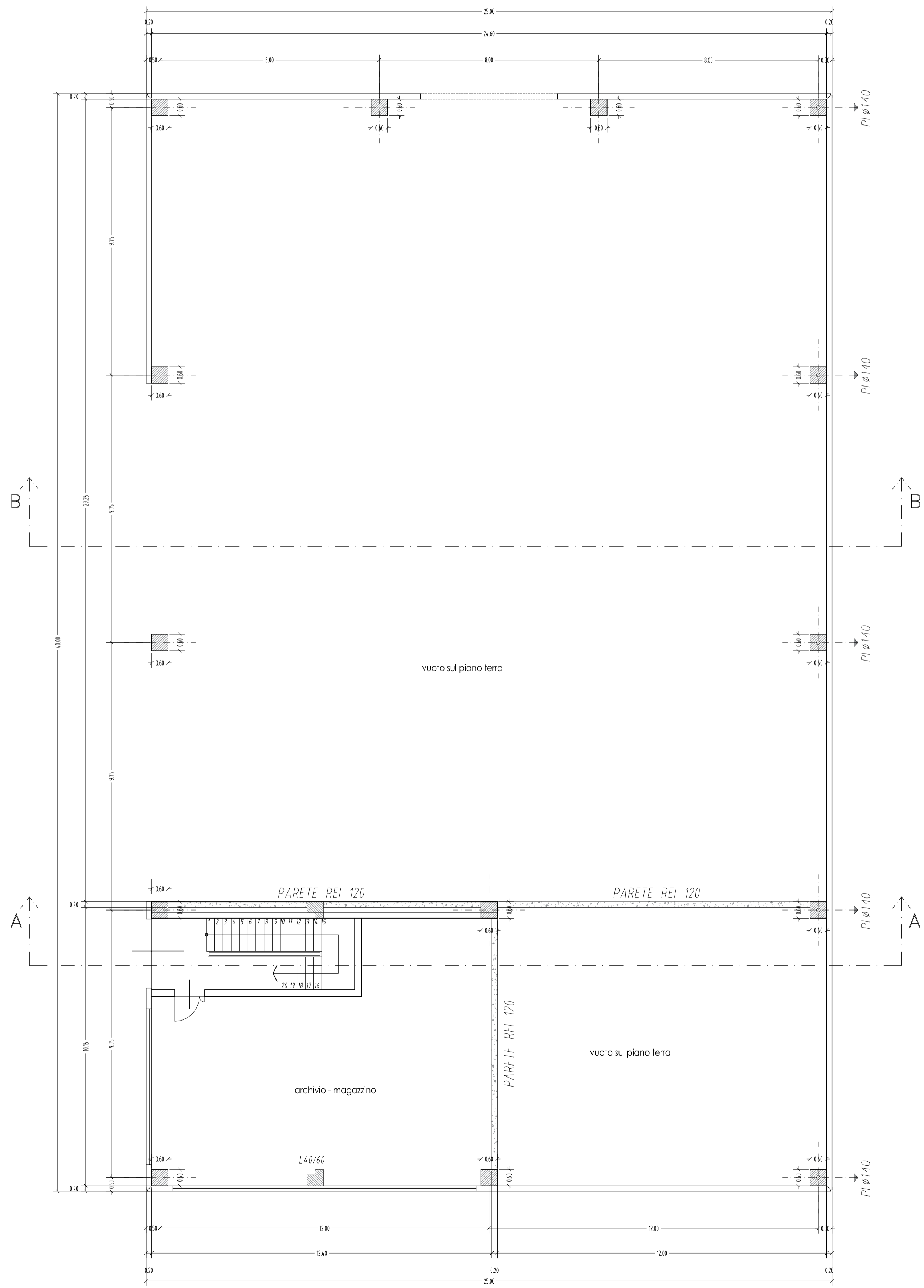
PIANO SECONDO - ARCHIVIO
