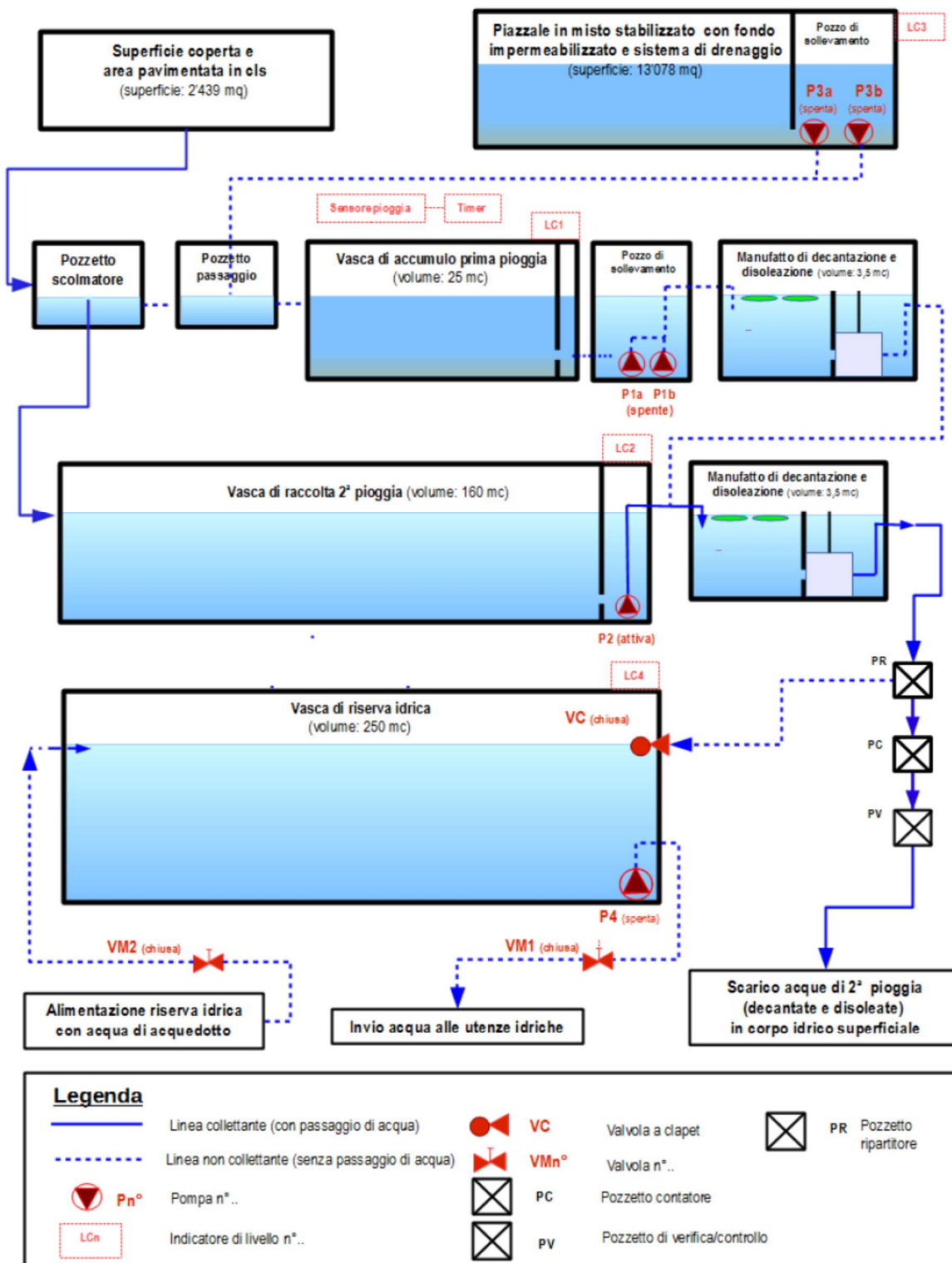
Figura 13: Sistema di raccolta, depurazione, riutilizzo e scarico acque.
