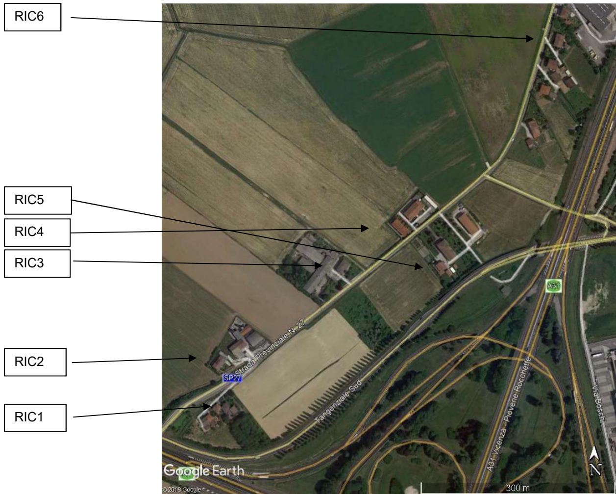
Figura 20: Individuazione dei recettori
