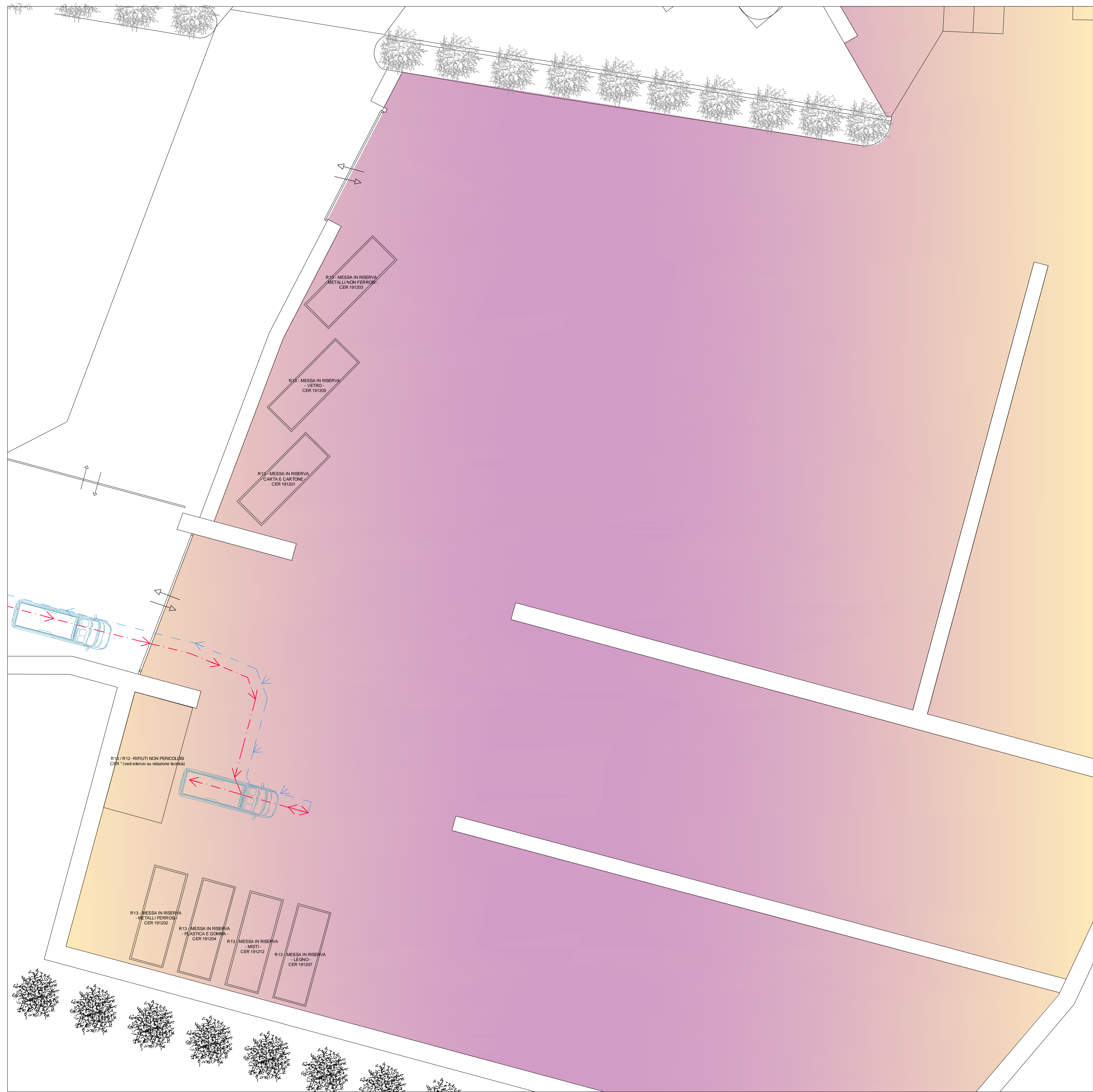
LAYOUT CASSONI PER MESSA IN RISERVA: METALLI FERROSI - PLASTICA E GOMMA - MISTI - LEGNO - CARTA E CARTONE - VETRO - METALLI NON FERROSI
