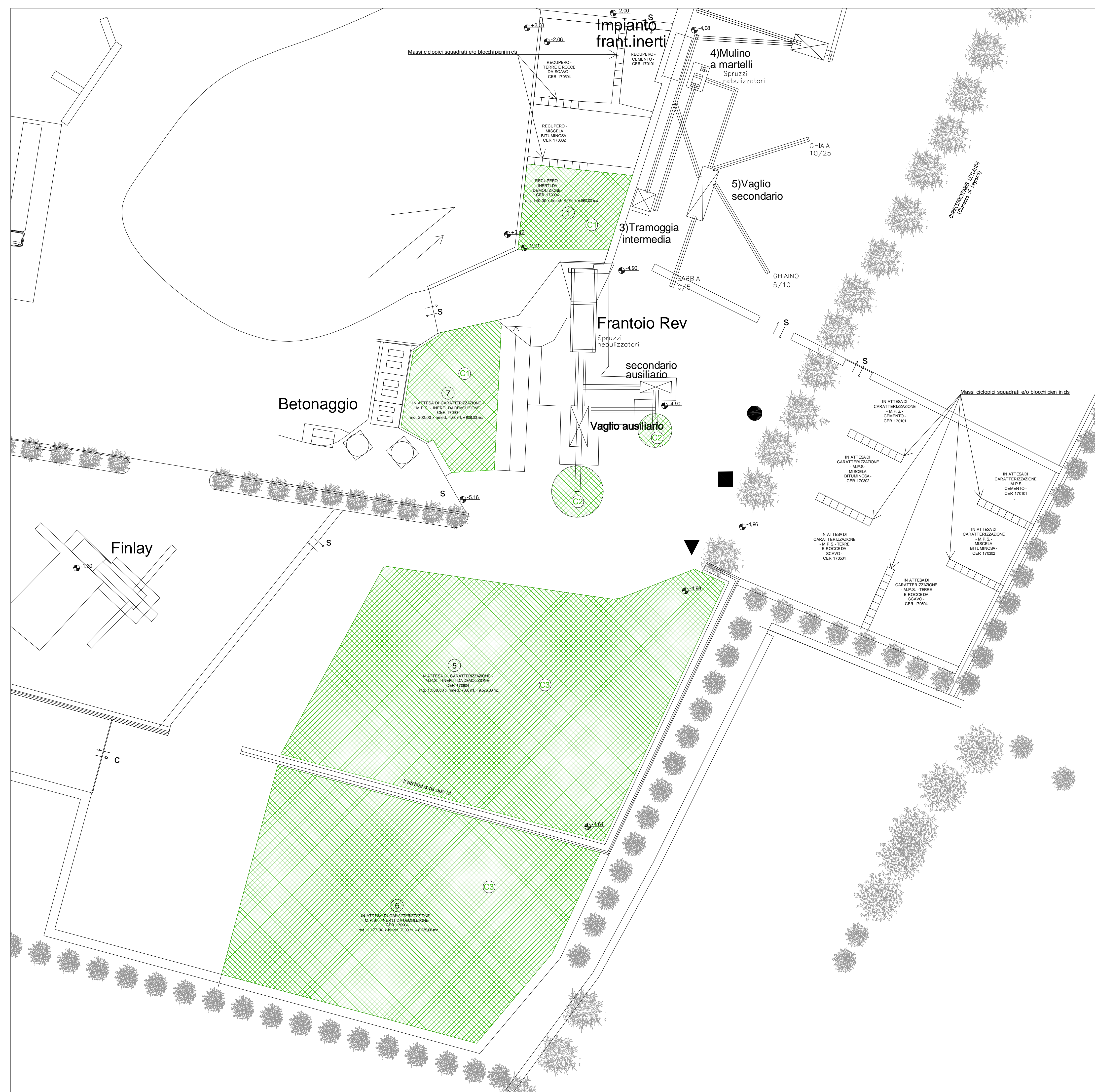
LAYOUT LINEA TRATTAMENTO A: FRANTUMAZIONE E/O VAGLIATURA INERTI DA DEMOLIZIONE - CER 170904:
