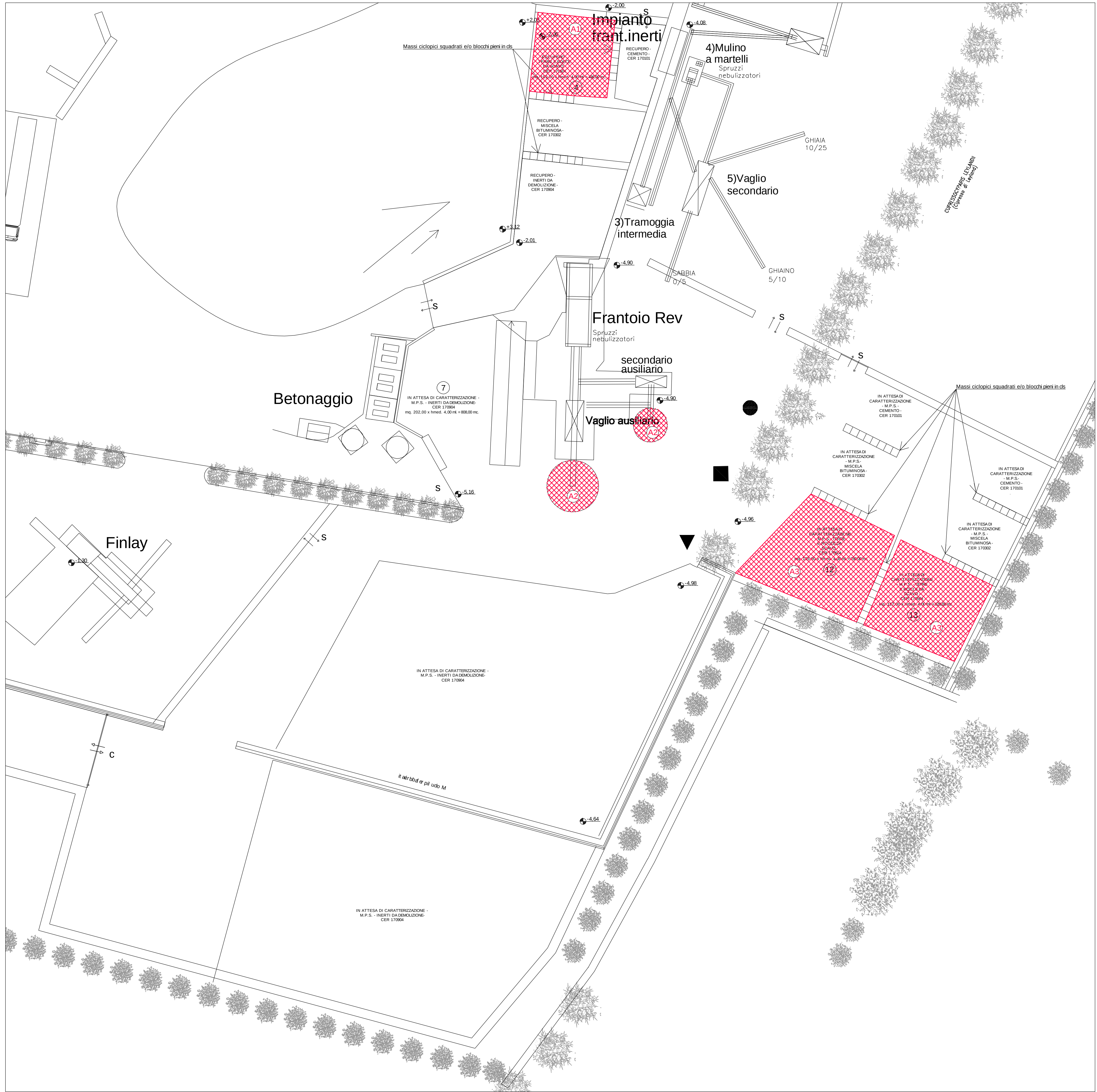
LAYOUT LINEA TRATTAMENTO A: FRANTUMAZIONE E/O VAGLIATURA TERRE E ROCCE DA SCAVO - CER 170504:
