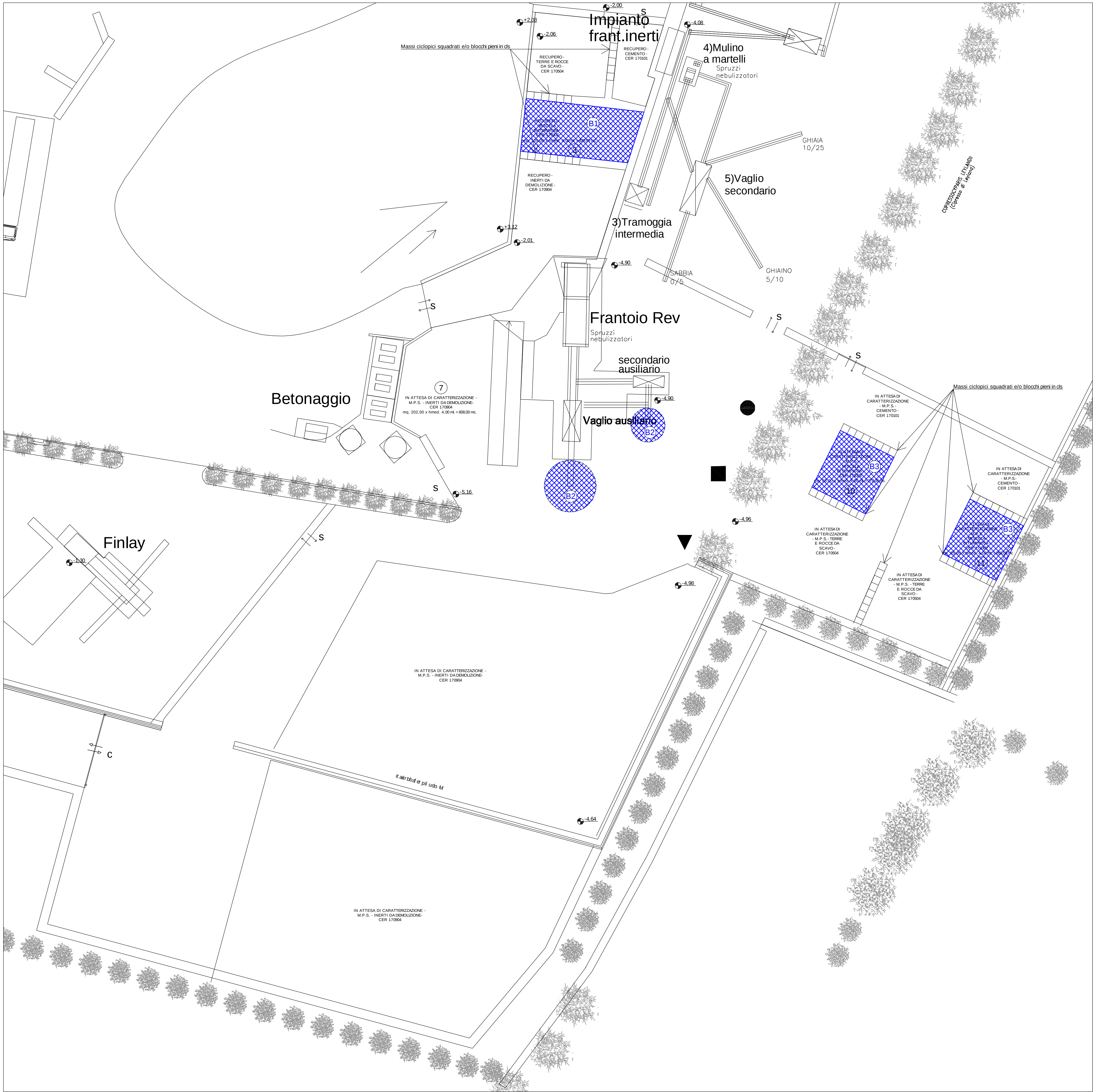
LAYOUT LINEA TRATTAMENTO A: FRANTUMAZIONE E/O VAGLIATURA MISCELE BITUMINOSE - CER 170302:
