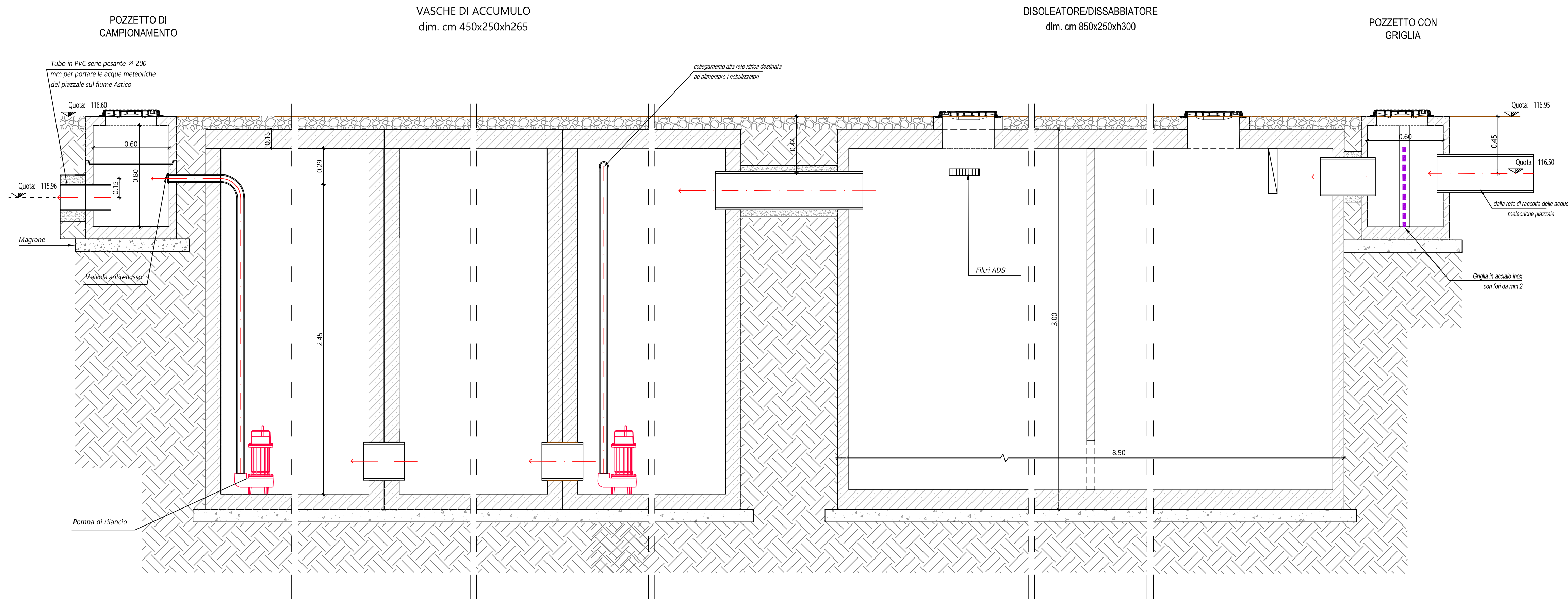
SEZIONE
