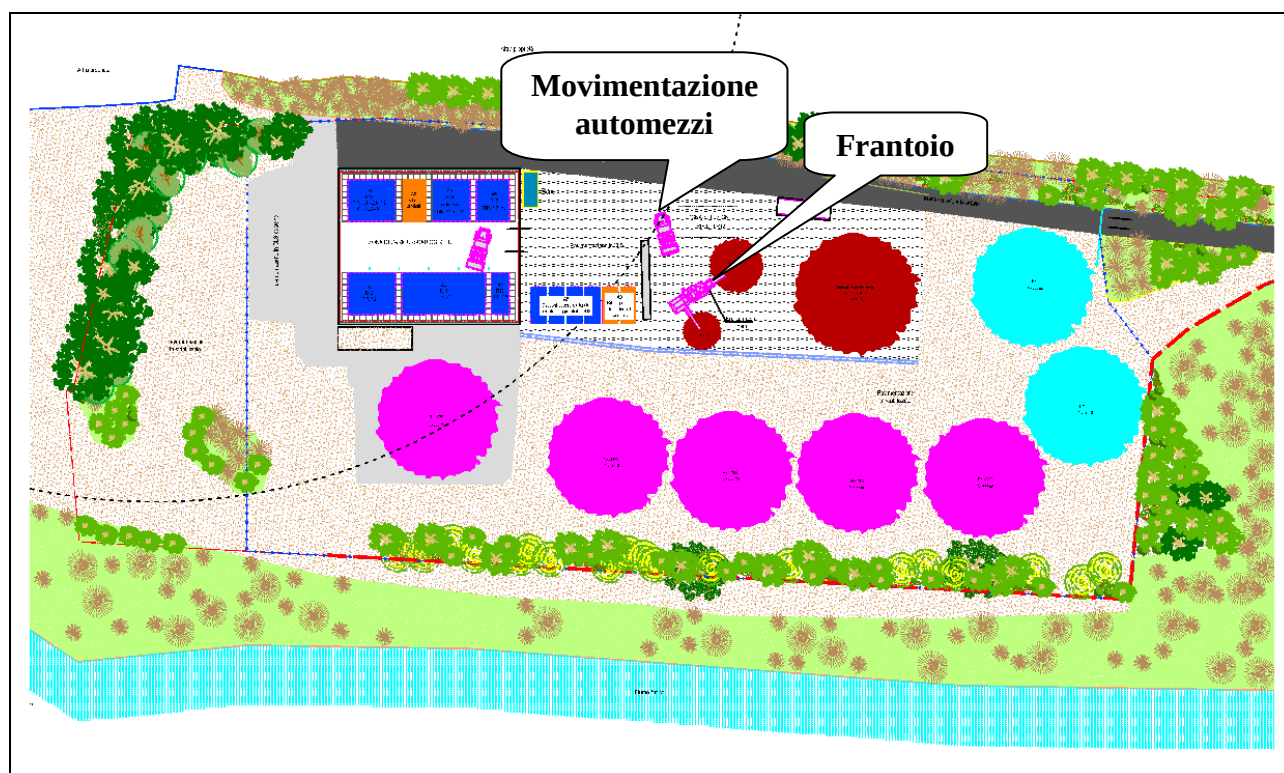
Fig. 2: layout produttivo allo stato futuro
