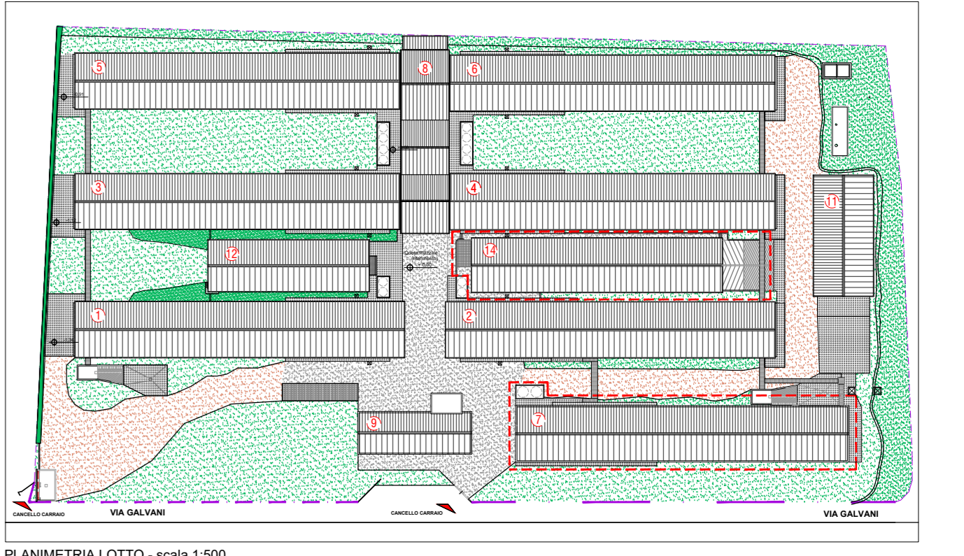
PLANIMETRIA LOTTO - scala 1:500
