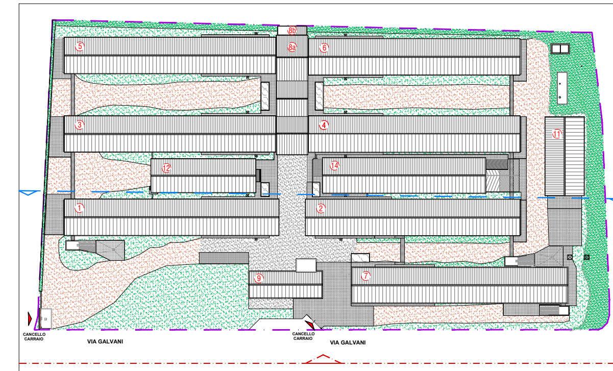
PLANIMETRIA DEGLI ESTERNI - SCALA 1:500
