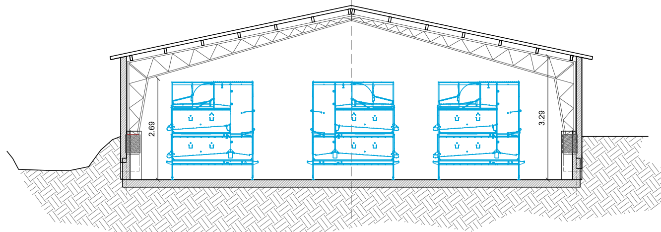
SEZIONE B-B Voliere
