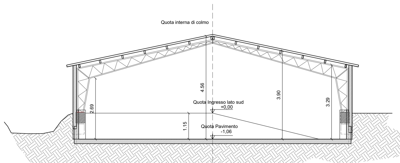
SEZIONE B-B
