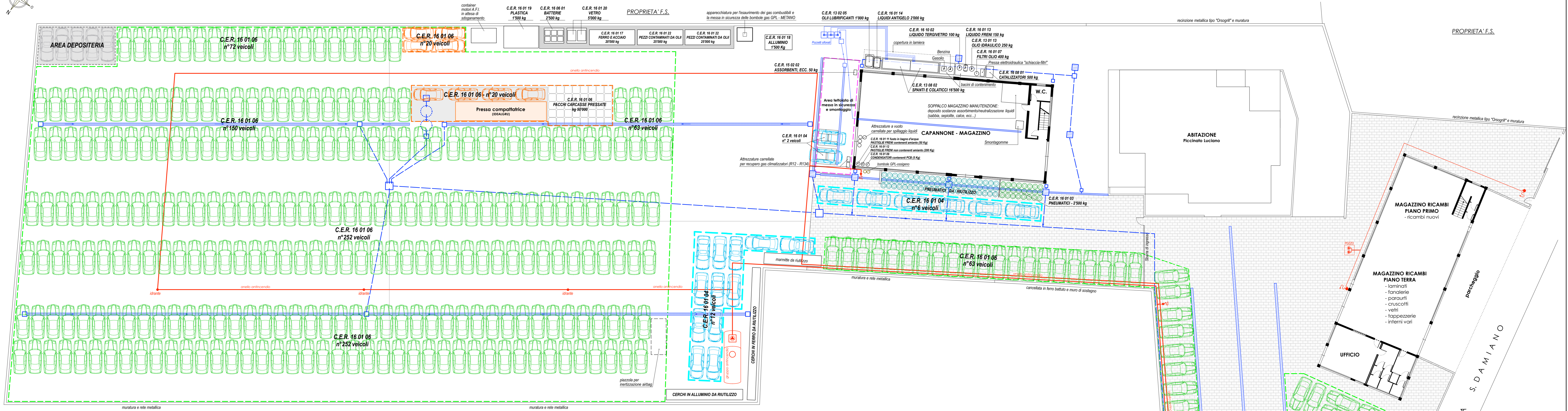
Planimetria / lay-out dell'impianto scala 1:200
