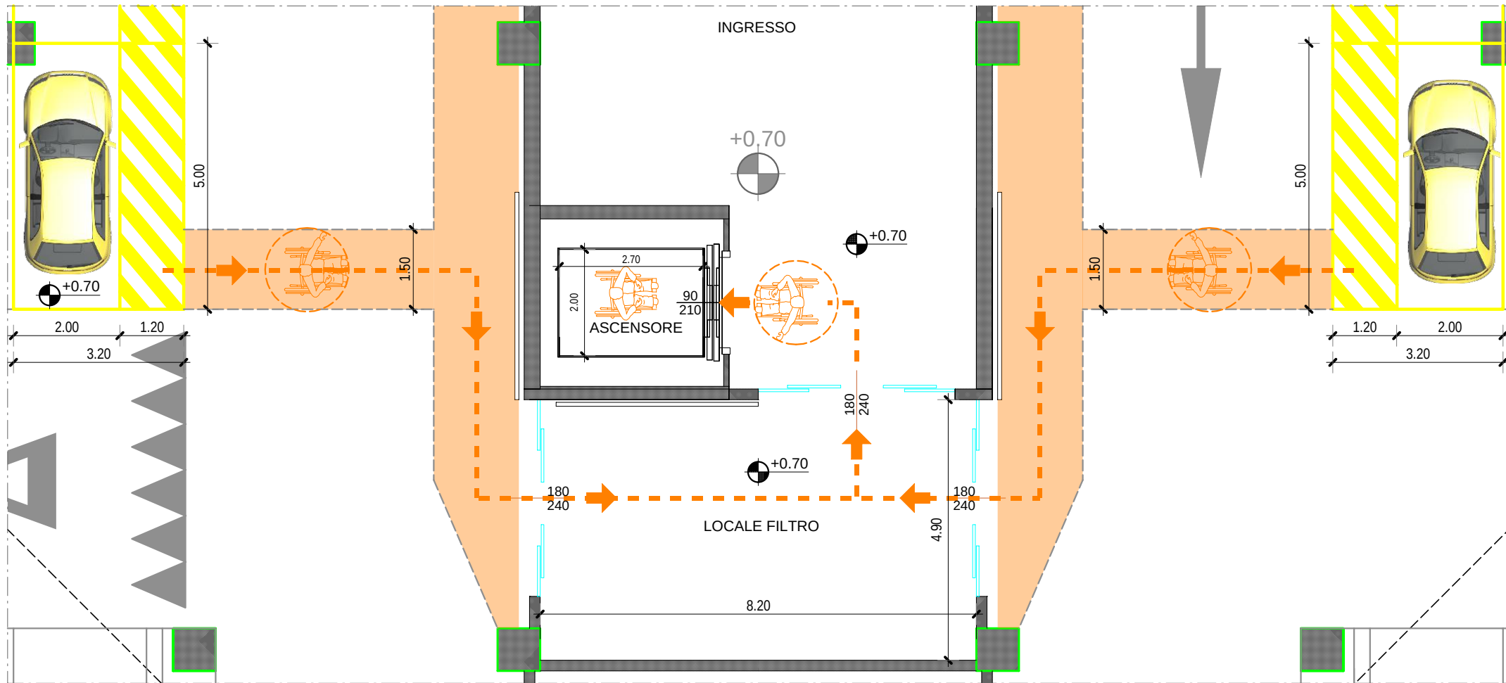
DIMOSTRAZIONE ACCESSIBILITA' DAL PIANO TERRA (PARCHEGGI) AL PIANO PRIMO (D.M. 236/89)
