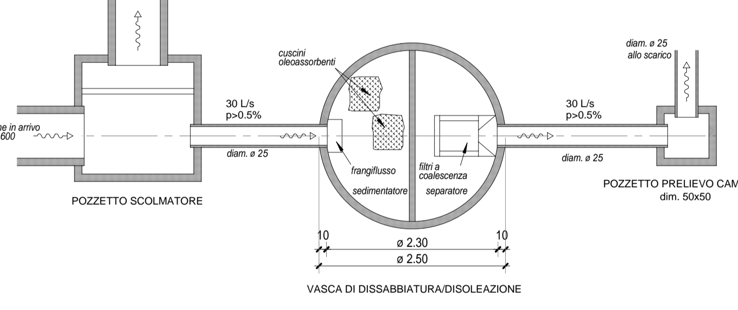
PROSPETTO SEZIONATO VASCHE scala 1:50
