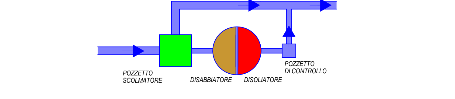
SCHEMA A BLOCCHI
