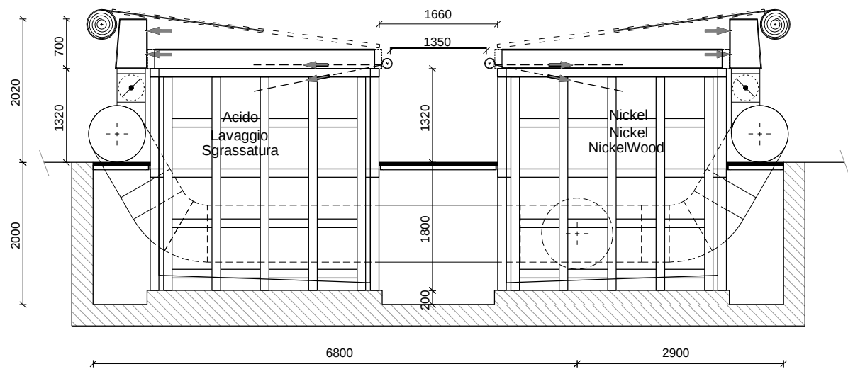
Sezionetrasversaleimpianto
