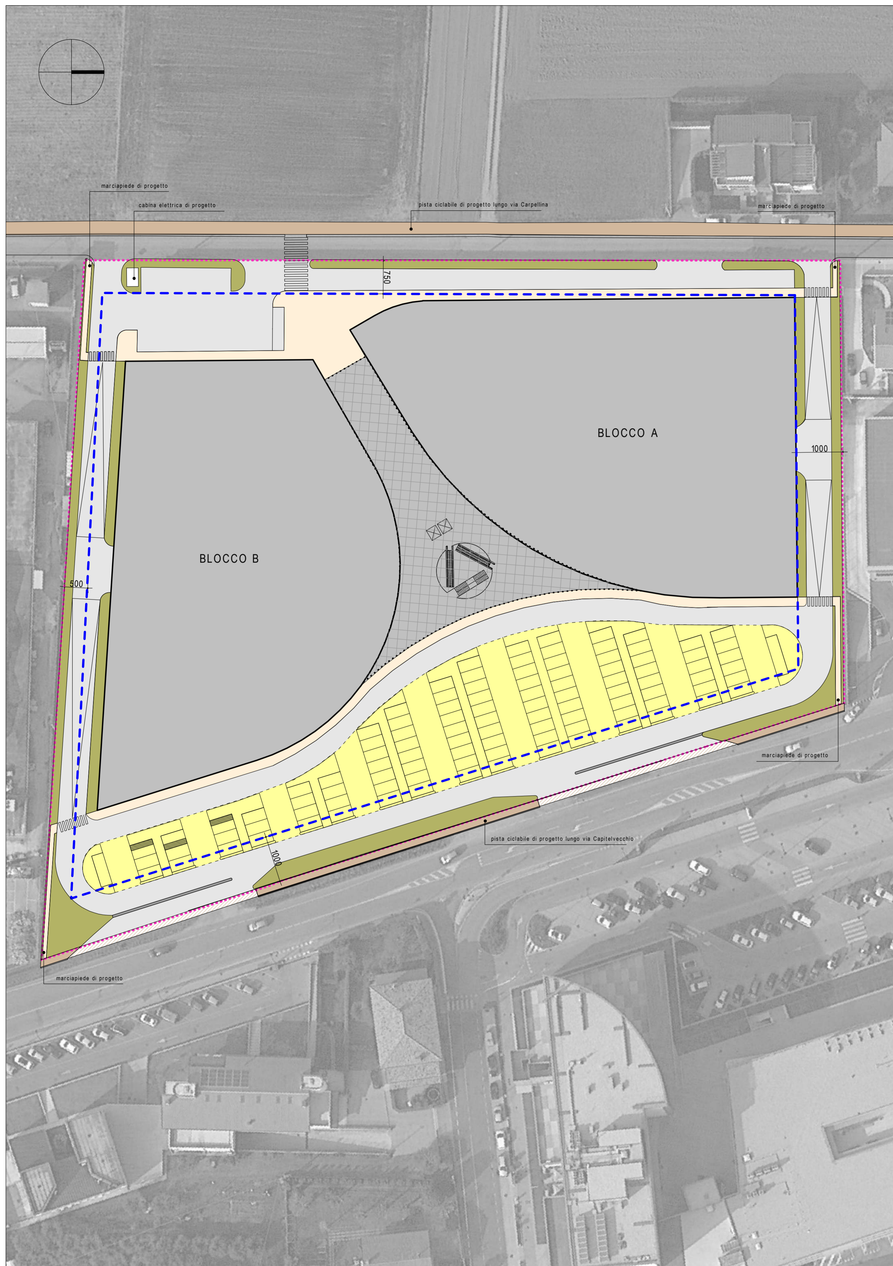
PLANIMETRIA CON INDICAZIONI PARAMETRI URBANISTICI ED AREE A DISPOSIZIONE - SCALA 1:500
