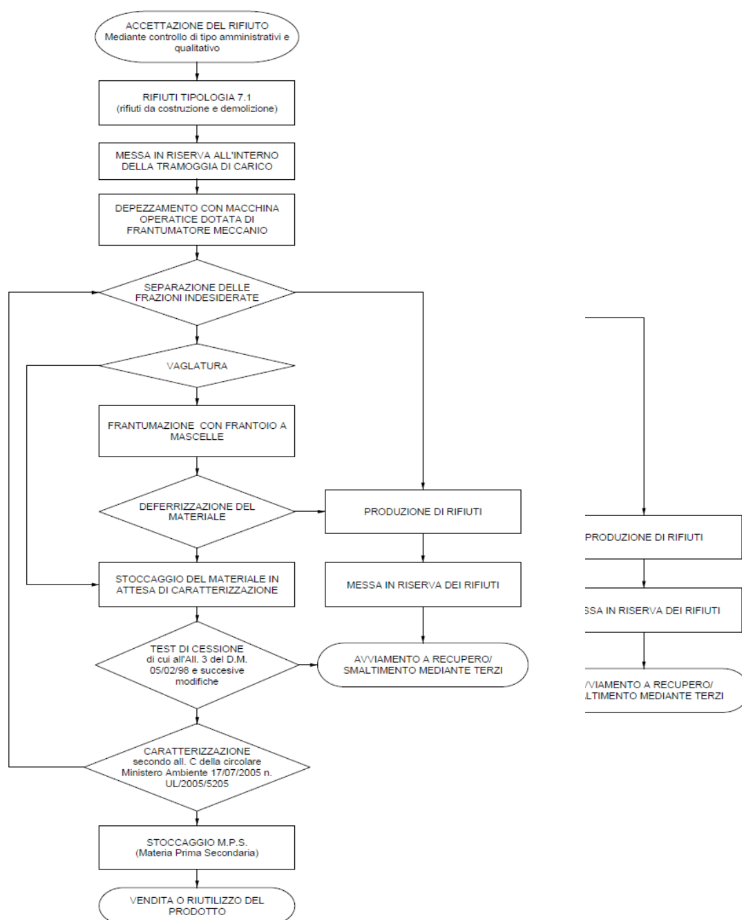
Schema a flusso per la tipologia 7.1
