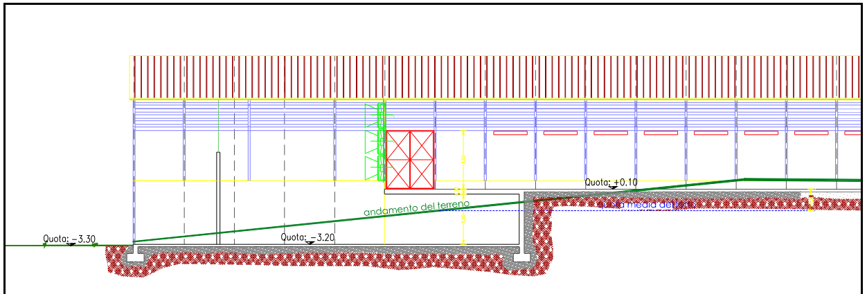
Sezione di progetto
