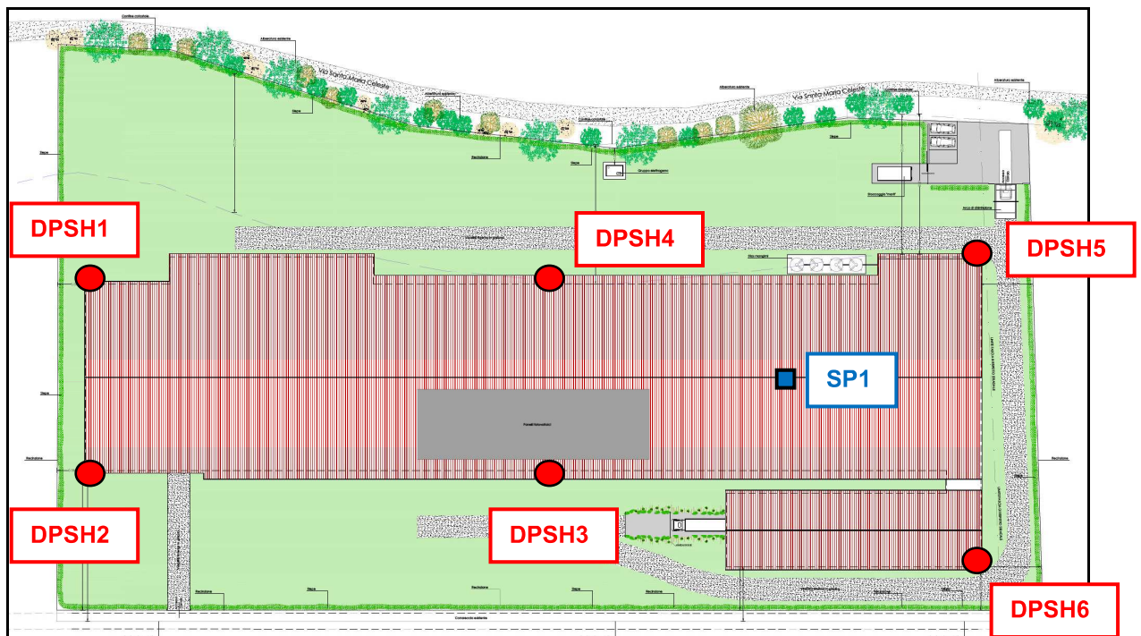
Planimetria di progetto con ubicazione delle indagini eseguite
